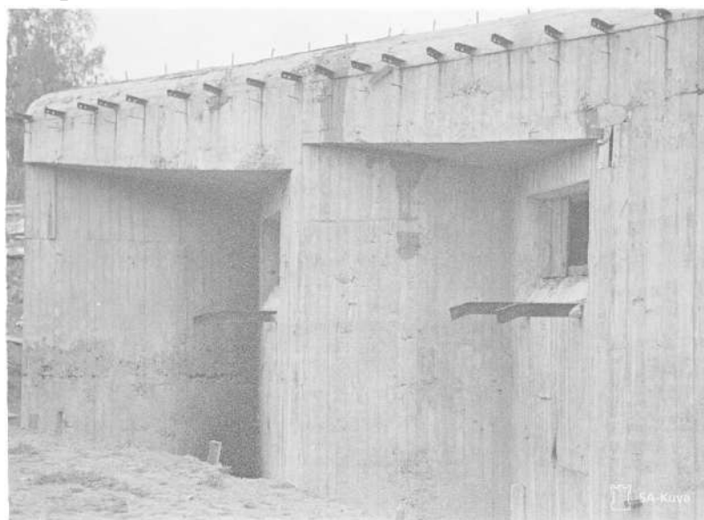
Советский полукапонир без вооружения, передовой рубеж Карельского укрепленного района в Раасули, Карельский перешеек. 1941 год, фото сделано финскими военными корреспондентами. sa-kiva.fi архив фотографий финских оборонительных сил
