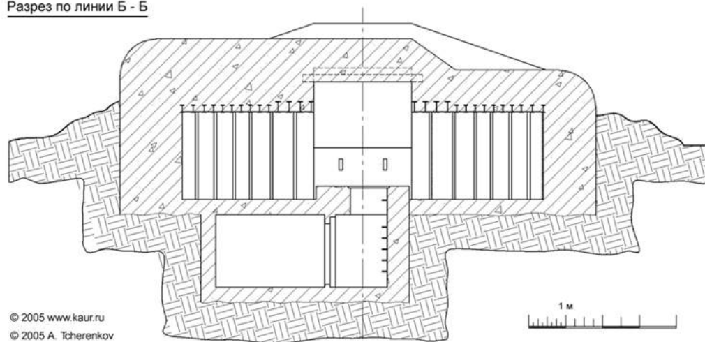
Разрез по линии Б - Б
