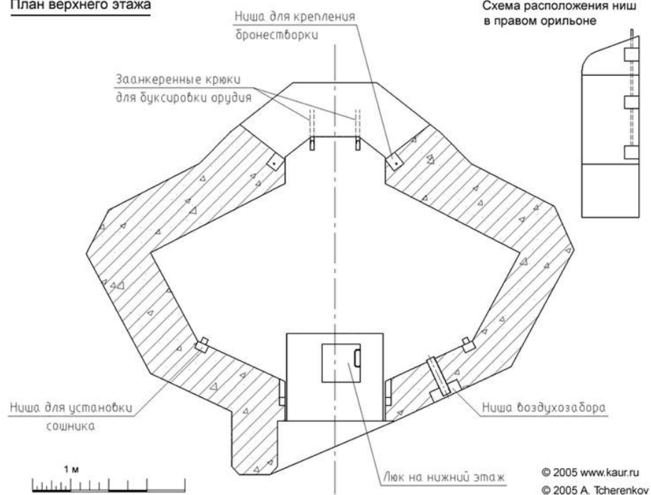
План верхнего этажа
