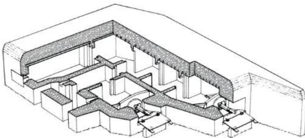
Схема полукапонира 1929-1930: фланговый огонь ведется в одну сторону https://topwar.ru/262328-artillerijskoe-vooruzhenie-https://topwar.ru
