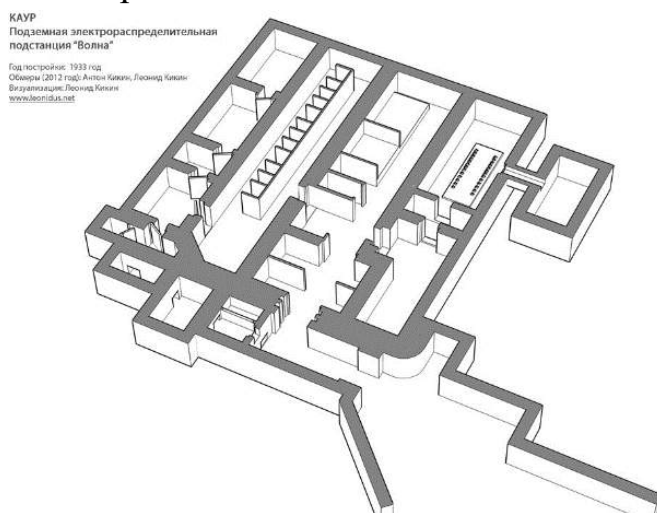
Подземная электростанция в Лемболово. 1933 г. Источник: https://www.aroundspb.ru
