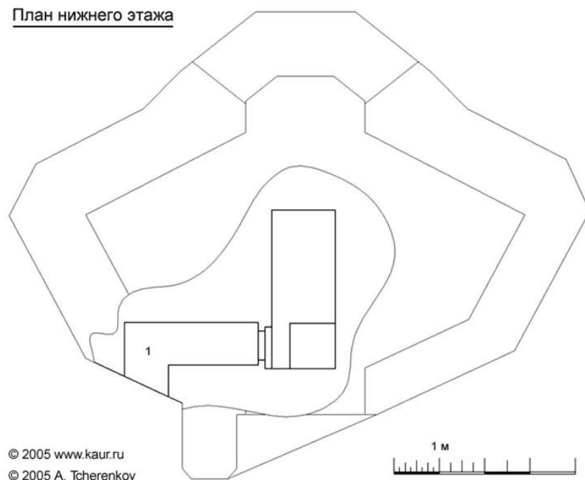
План нижнего этажа. Цифрой 1 обозначен эвакуационный выход с нижнего этажа. Источник: https://www.kaur.ru
