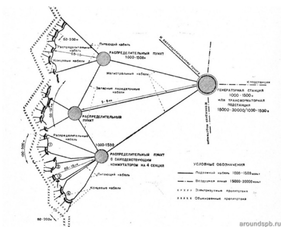
Схема сети питающих проводов (на примере Лемболовского батрайона). 1938 год.
