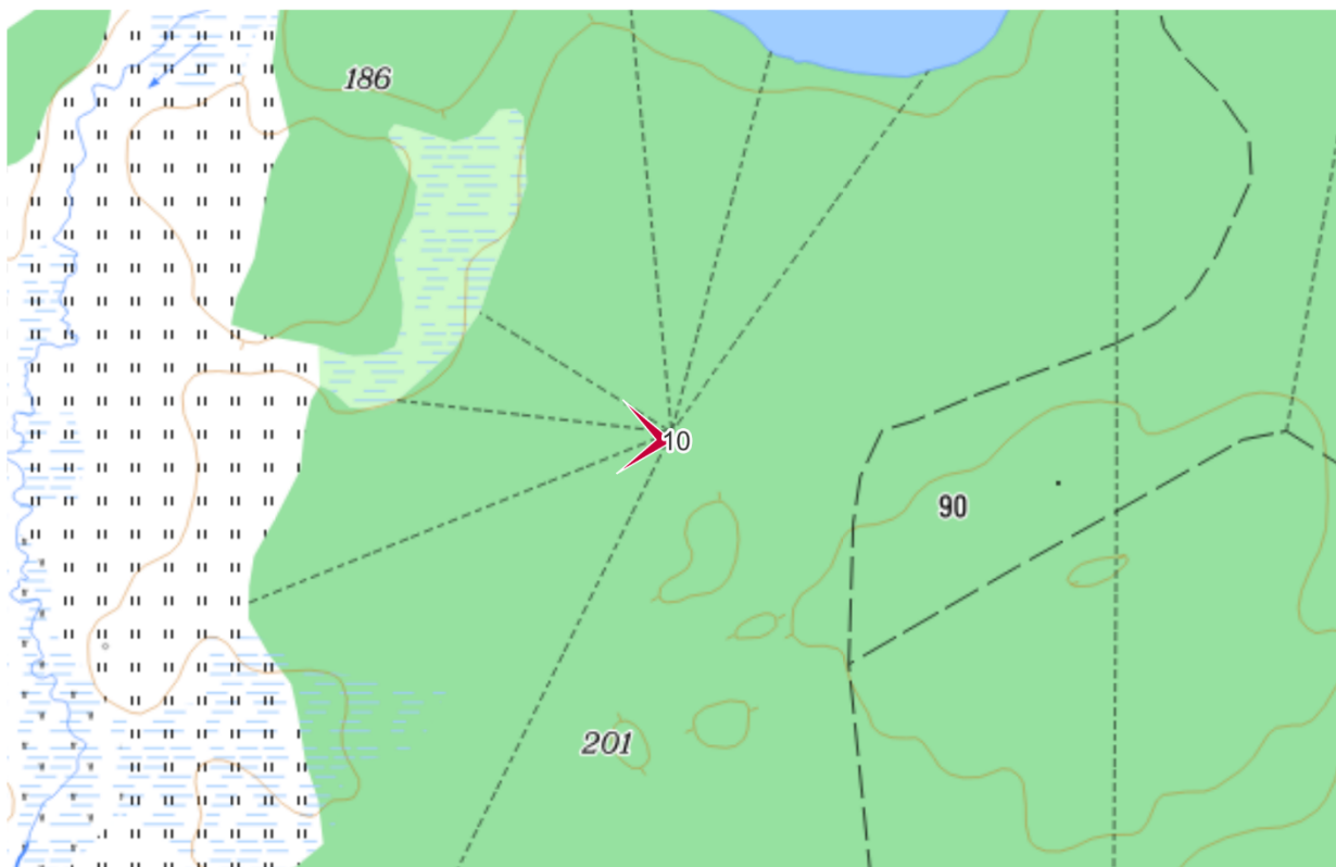
Фото 10. Выявленный объект культурного наследия «Карельский укрепленный район. Перемякский батальонный район обороны. ДОТ № 824. Пулеметная огневая точка». Направление съемки запад.
