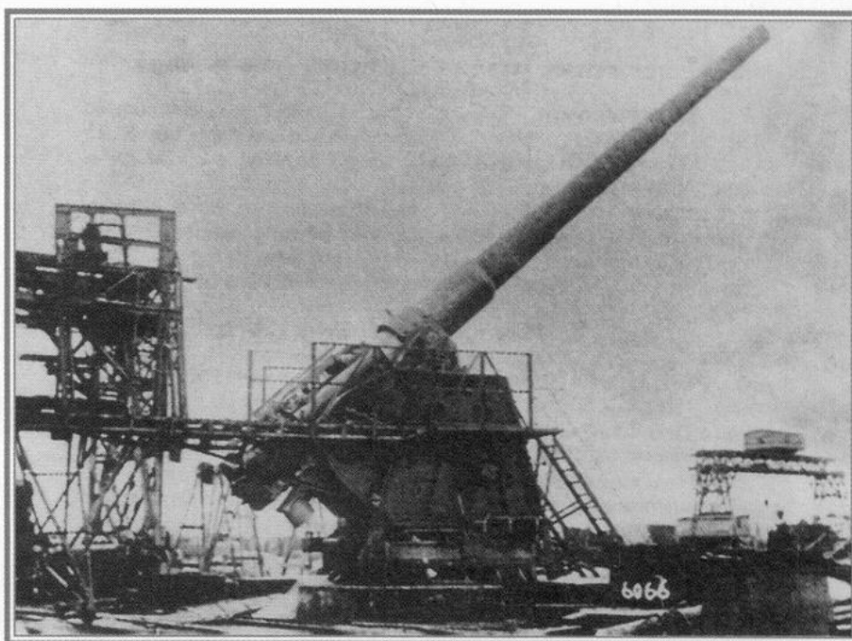
356-мм орудие 52 калибра длиной на Морском полигоне (НИМАП). 1920-е гг.
