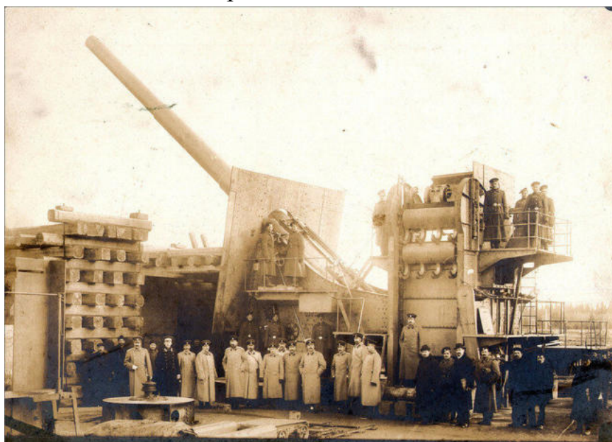
12-дм. в 52 калибра орудие на лафете конструкции Р. А. Дурлахера. Главный артиллерийский полигон. Не ранее 1910 г. Источник: Война и оружие. Труды пятой Международной научно-практической конференции. Ч. 1. СПб.: ВИМАИВиВС, 2014.
