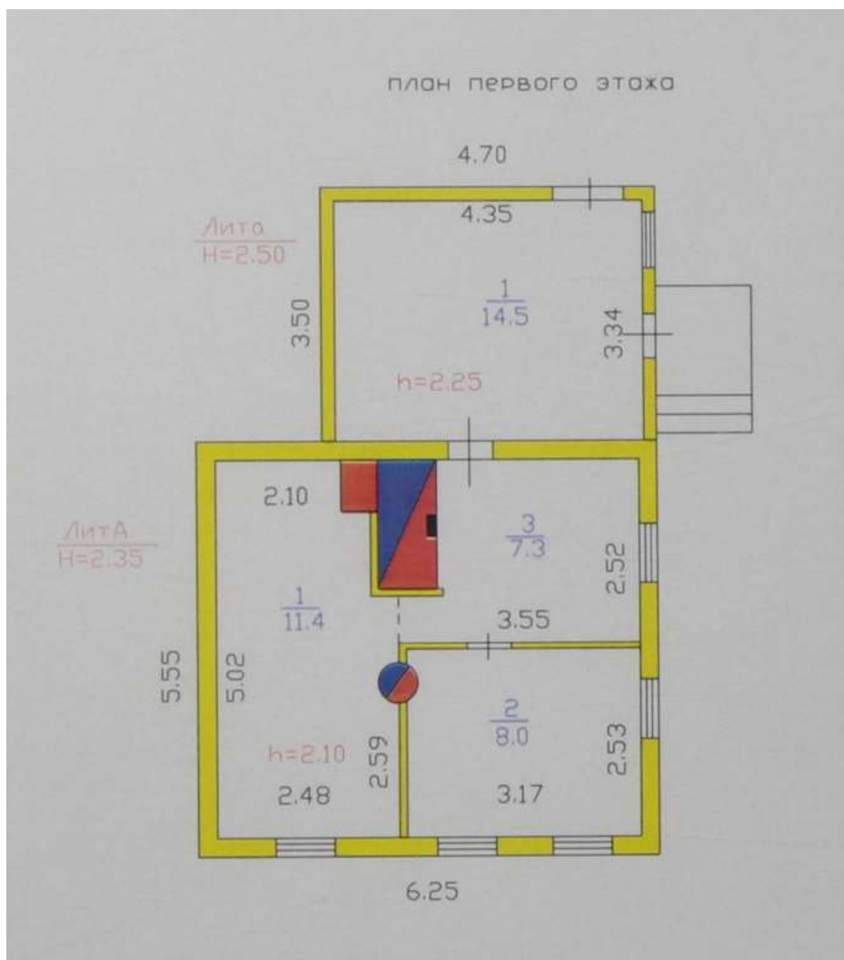
Рис. 12. Поэтажный план на индивидуальный жилой дом № 28 по ул. Центральная дер. Лампово. 12
