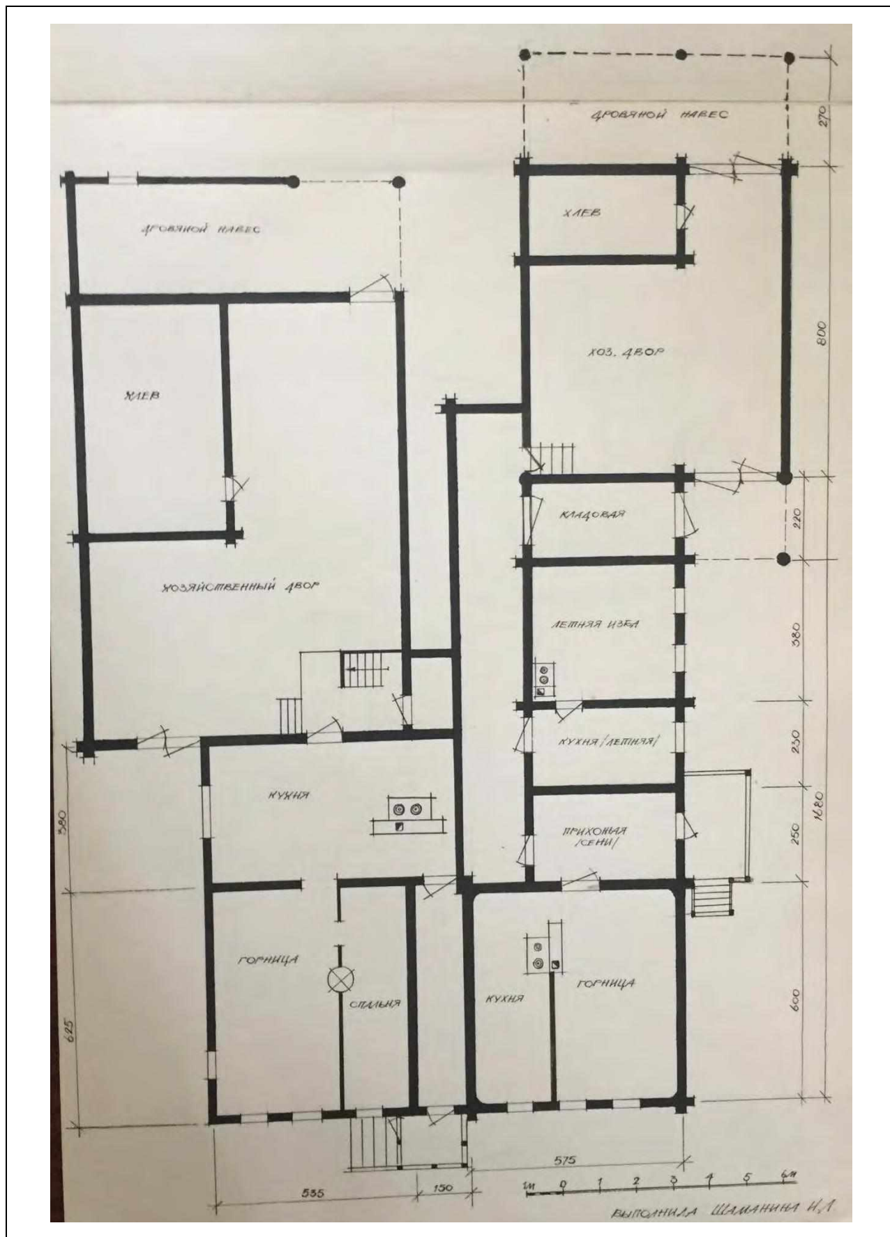
15. Историческая среда. План дома по адресу ул. Жуковка, 11 (рисунок). Ф. 1641, д. 1641-21.
