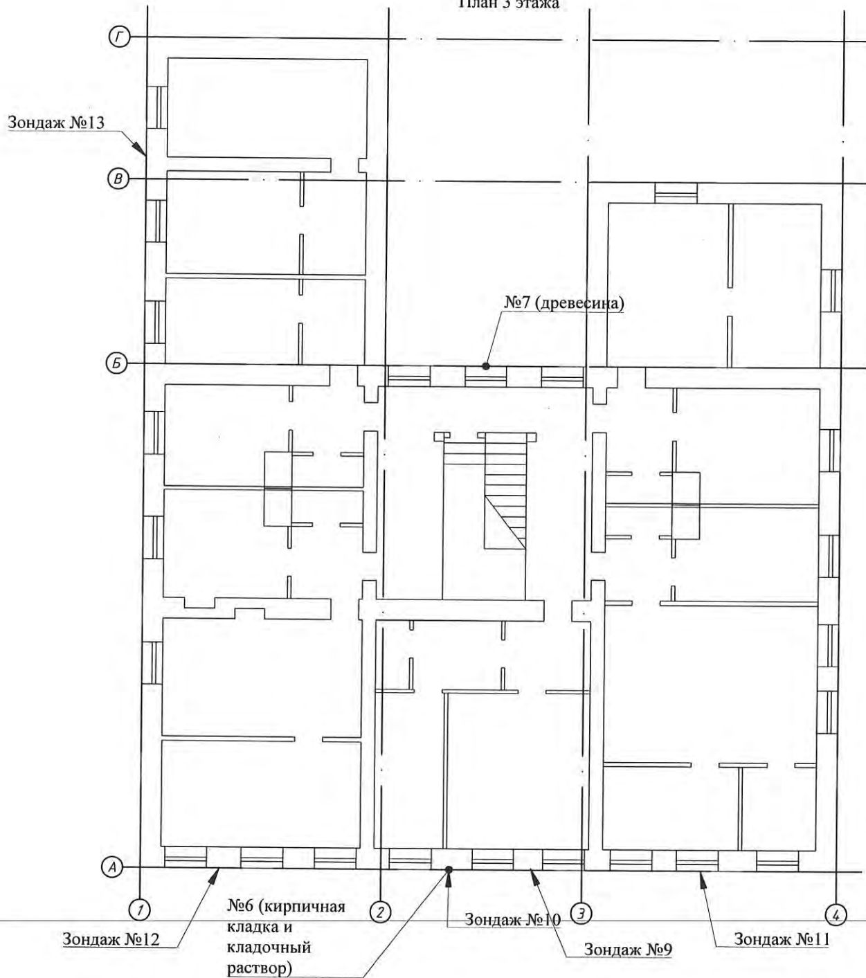
План 3 этажа
