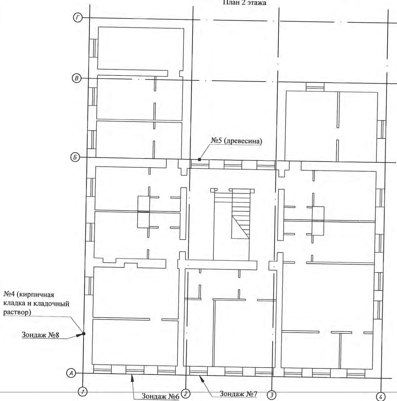
План 2 этажа
