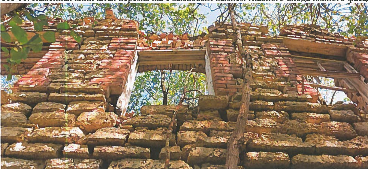
Фото 17. Вид на оконные проемы южного фасада. Обрамлены кирпичной кладкой. Заполнения оконных проемов утрачены.
