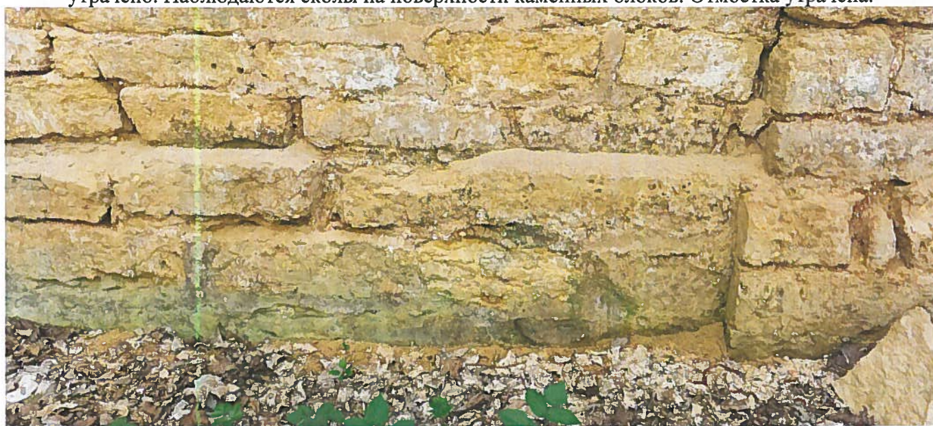
Фото 2. Вид на цоколь. Материал цоколя – обработанные каменные блоки. Шовное заполнение утрачено. Отмостка утрачена.
