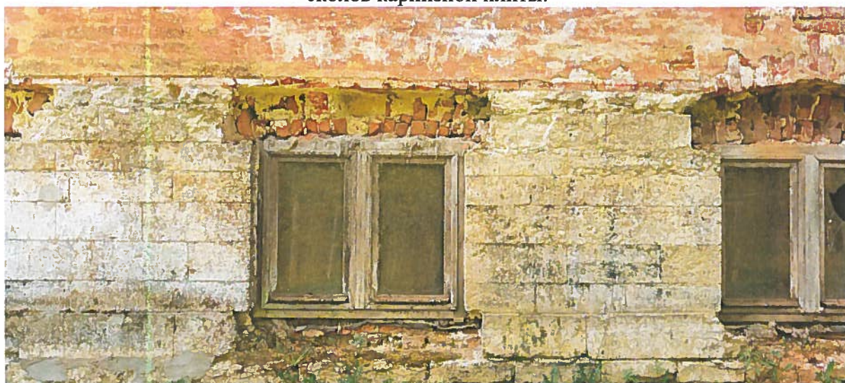
Фото 4. Фрагмент северного фасада. Вид на цокольный этаж. Наблюдается утрата кирпичных клинчатых перемычек оконных проемов.
