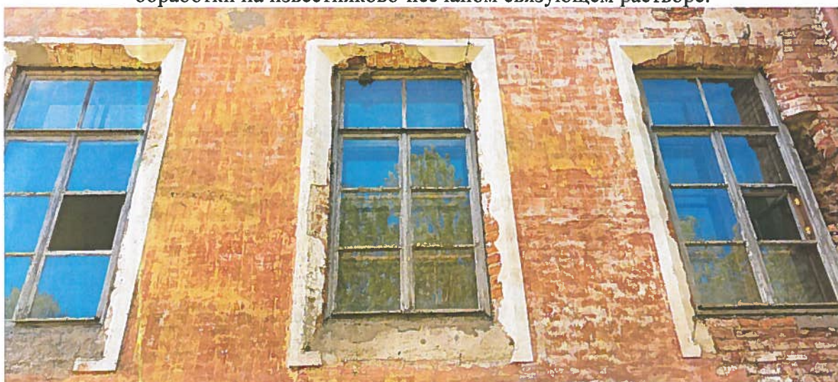
Фото 11. Фрагмент северного фасада. Оконные проемы двухэтажного объема. Наблюдаются вывалы кирпичей.
