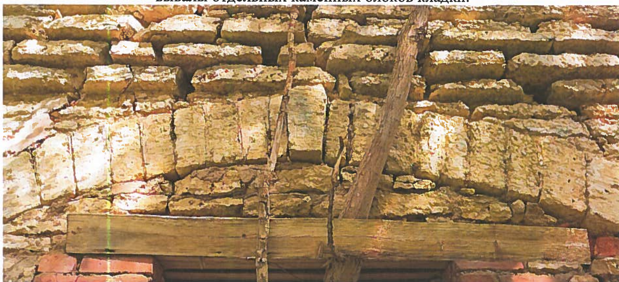
Фото 16. Каменная клинчатая перемычка с замковым камнем главного входа южного фасада.
