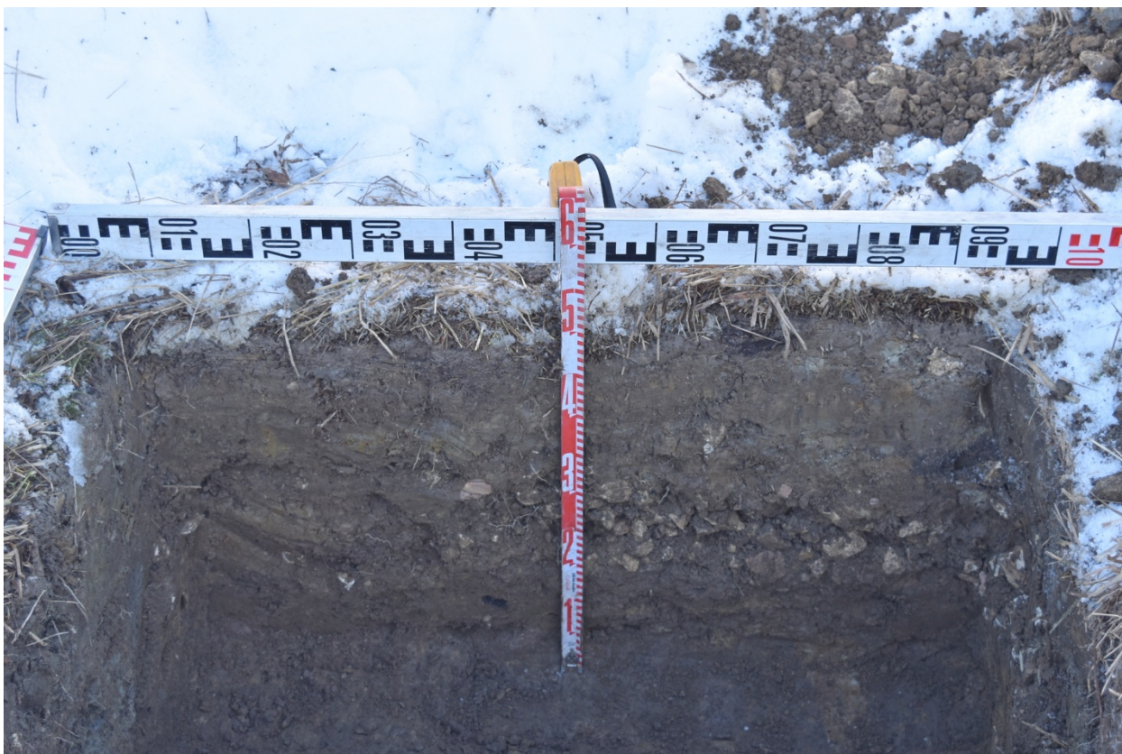
Рис. 64. Ленинградская обл., Ломоносовский р-н, Низино-2026. Стратиграфия шурфа 3 (северная стенка) и прокоп материка. Вид с юга.
