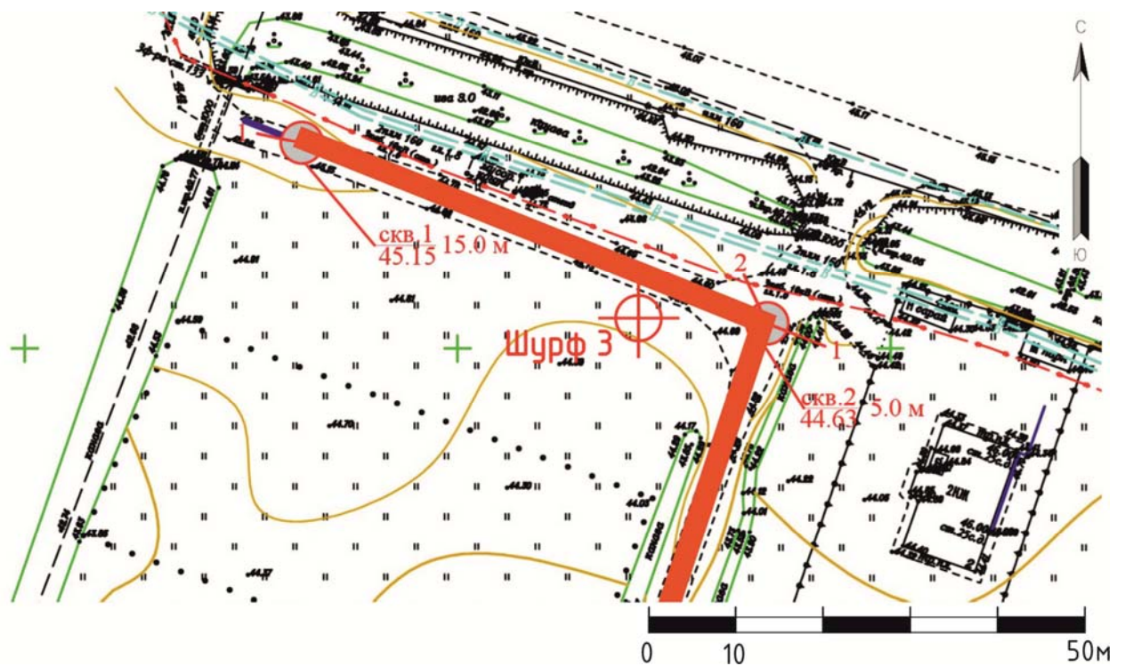
Рис. 60. Ленинградская обл., Ломоносовский р-н, Низино – 2026. Расположение шурфа 3 на топоплане, предоставленном Заказчиком.
