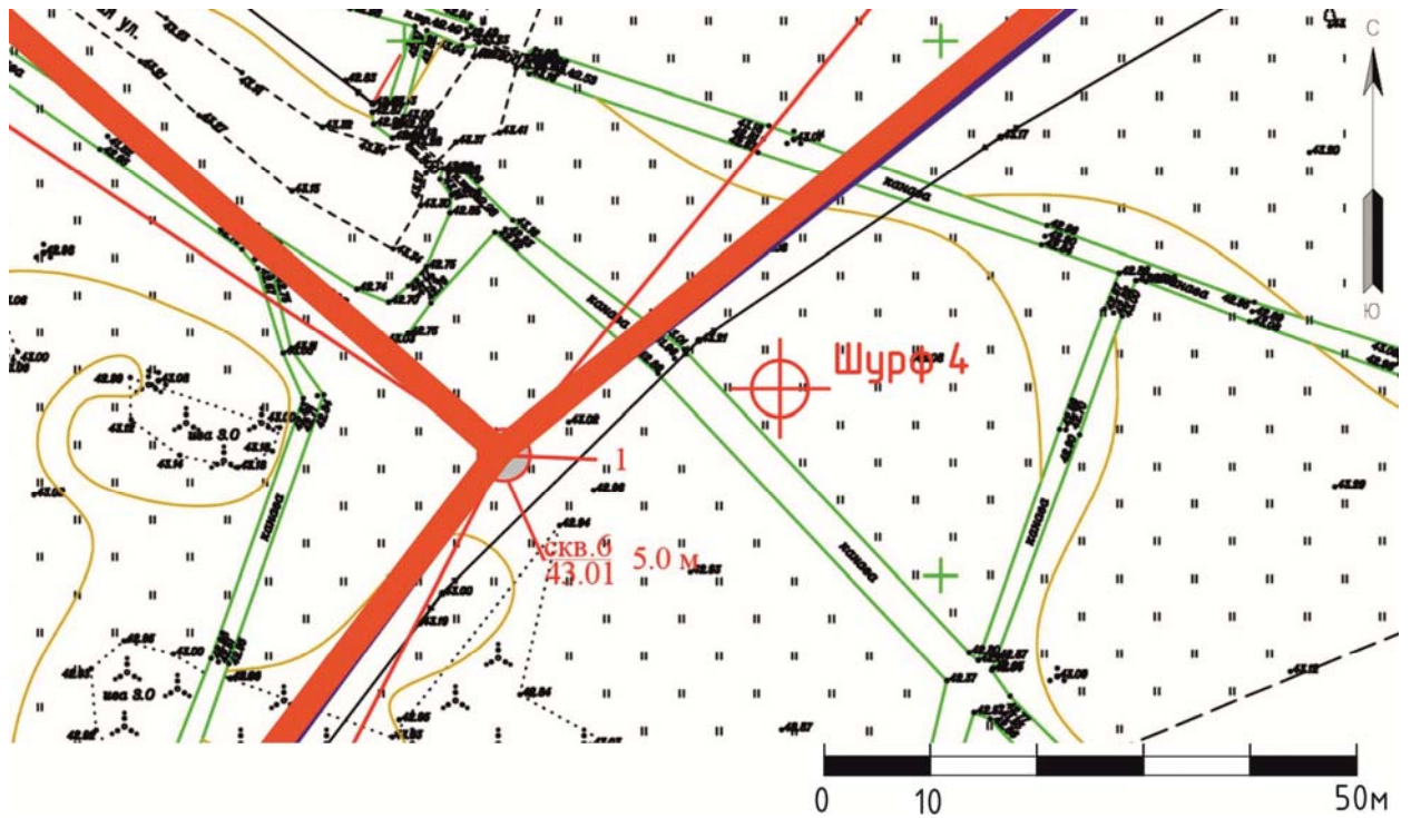
Рис. 66. Ленинградская обл., Ломоносовский р-н, Низино – 2026. Расположение шурфа 4 на топоплане, предоставленном Заказчиком.
