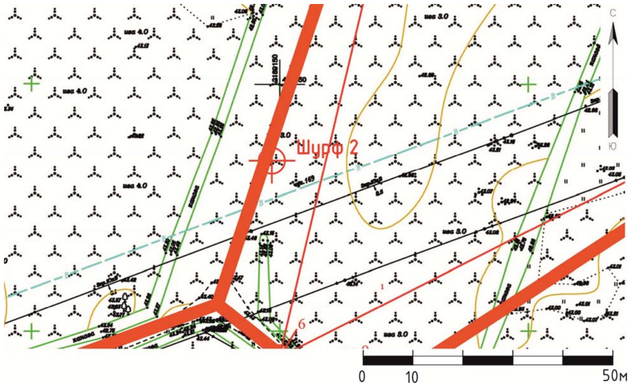
Рис. 54. Ленинградская обл., Ломоносовский р-н, Низино – 2026. Расположение шурфа 2 на топоплане, предоставленном Заказчиком.
