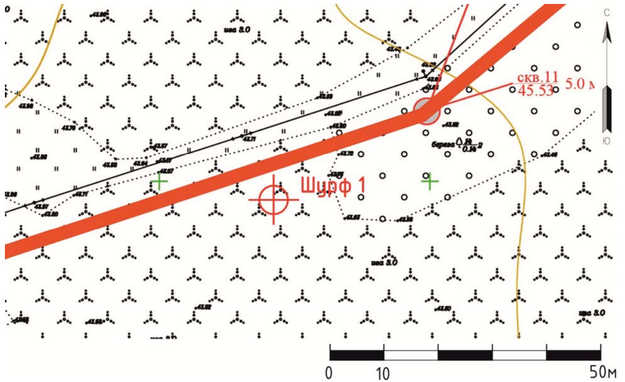
Рис. 48. Ленинградская обл., Ломоносовский р-н, Низино – 2026. Расположение шурфа 1 на топоплане, предоставленном Заказчиком.
