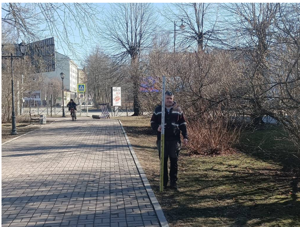
Фото 1. «Наружный газопровод до границ земельного участка, расположенного по адресу: Российская Федерация, Ленинградская область, муниципальный район Выборгский, г. Выборг, ул. Подгорная, д. 14/7 (47:01:0107001:2957). Точка фотофиксации 1. Общий вид на трассу проектируемого газопровода с СЗ.
