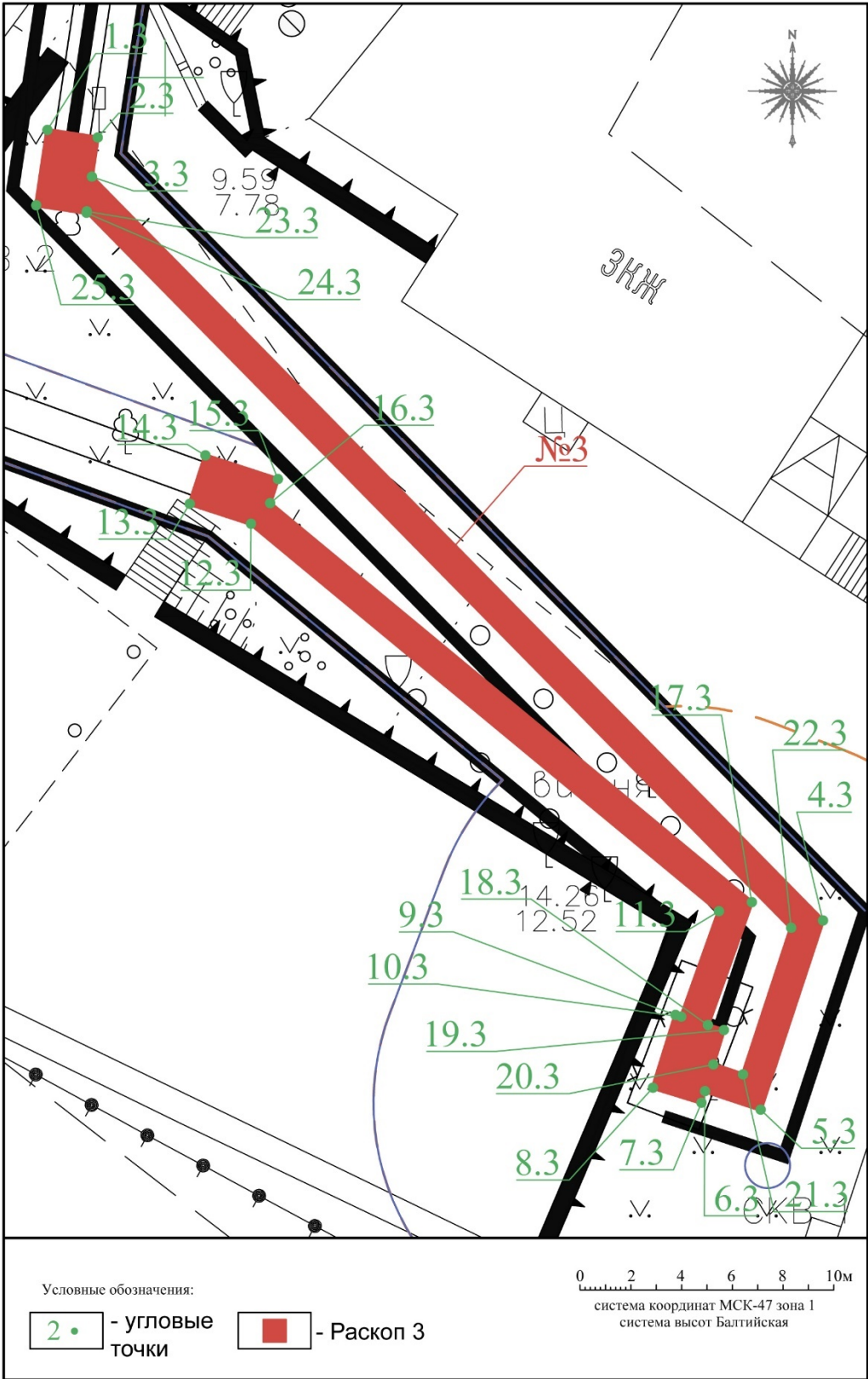
11. План проекта проведения археологических работ на территории ОК(А)Н «Культурный слой средневекового Выборга». Раскопы 2 и 3.
