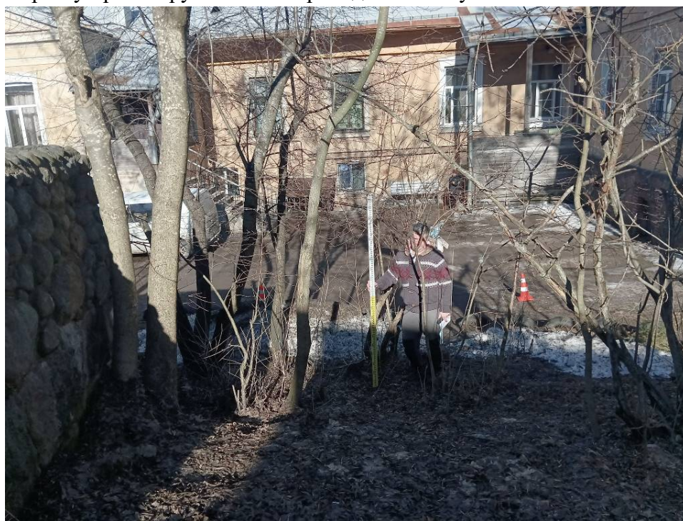
Фото 38. «Наружный газопровод до границ земельного участка, расположенного по адресу: Российская Федерация, Ленинградская область, муниципальный район Выборгский, г. Выборг, ул. Подгорная, д. 14/7 (47:01:0107001:2957). Точка фотофиксации 15. Общий вид на трассу проектируемого газопровода с ЮЮЗ.
