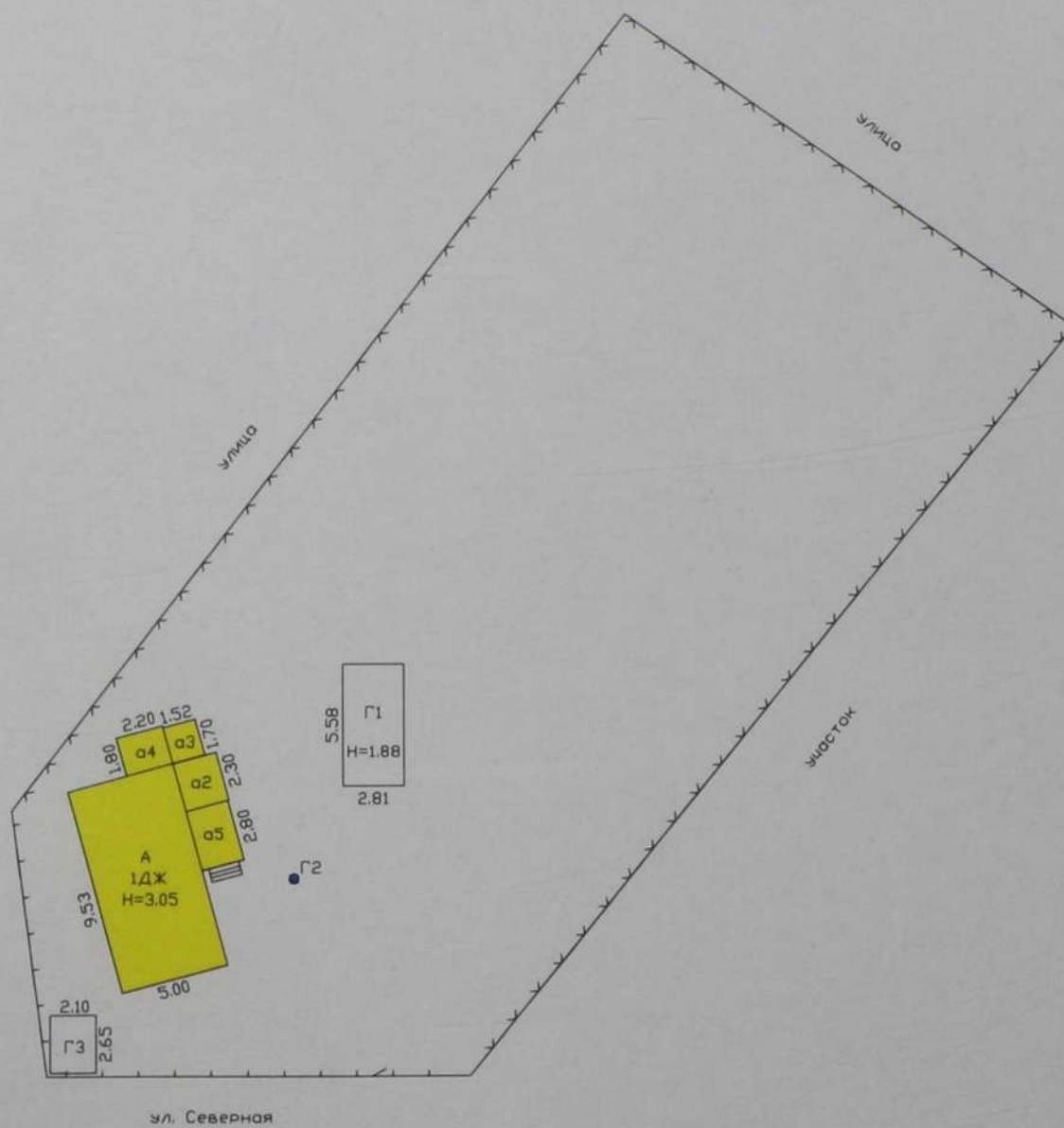
схема земельного участка
