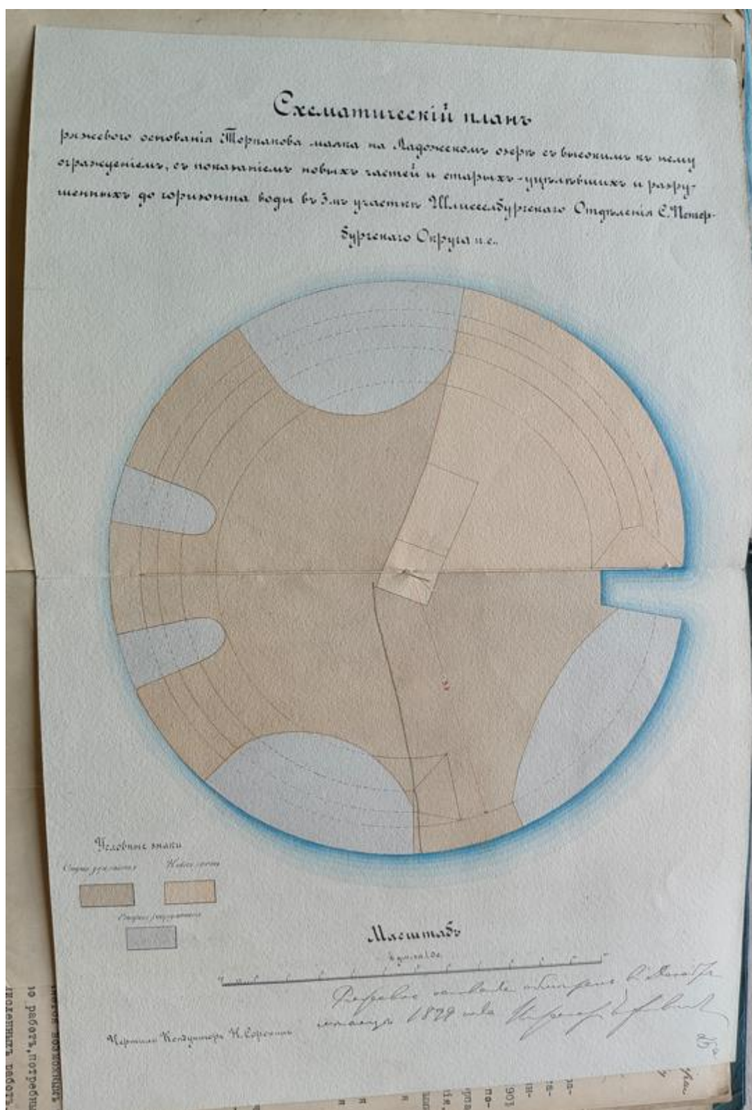
Илл. 20. Схематичный план ряжевого основания Торпакова маяка с показанием старых, новых и разрушенных частей. 1899 г. (источник: ЦГИА СПб. Ф. 921. Оп. 95. Д. 1962).
