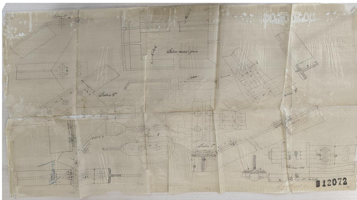
Илл. 24. Громоотвод для Торпакова маяка в Ладожском озере. 1897 г. (источник: ЦГИА СПб. Ф. 921. Оп. 95. Д. 502).
