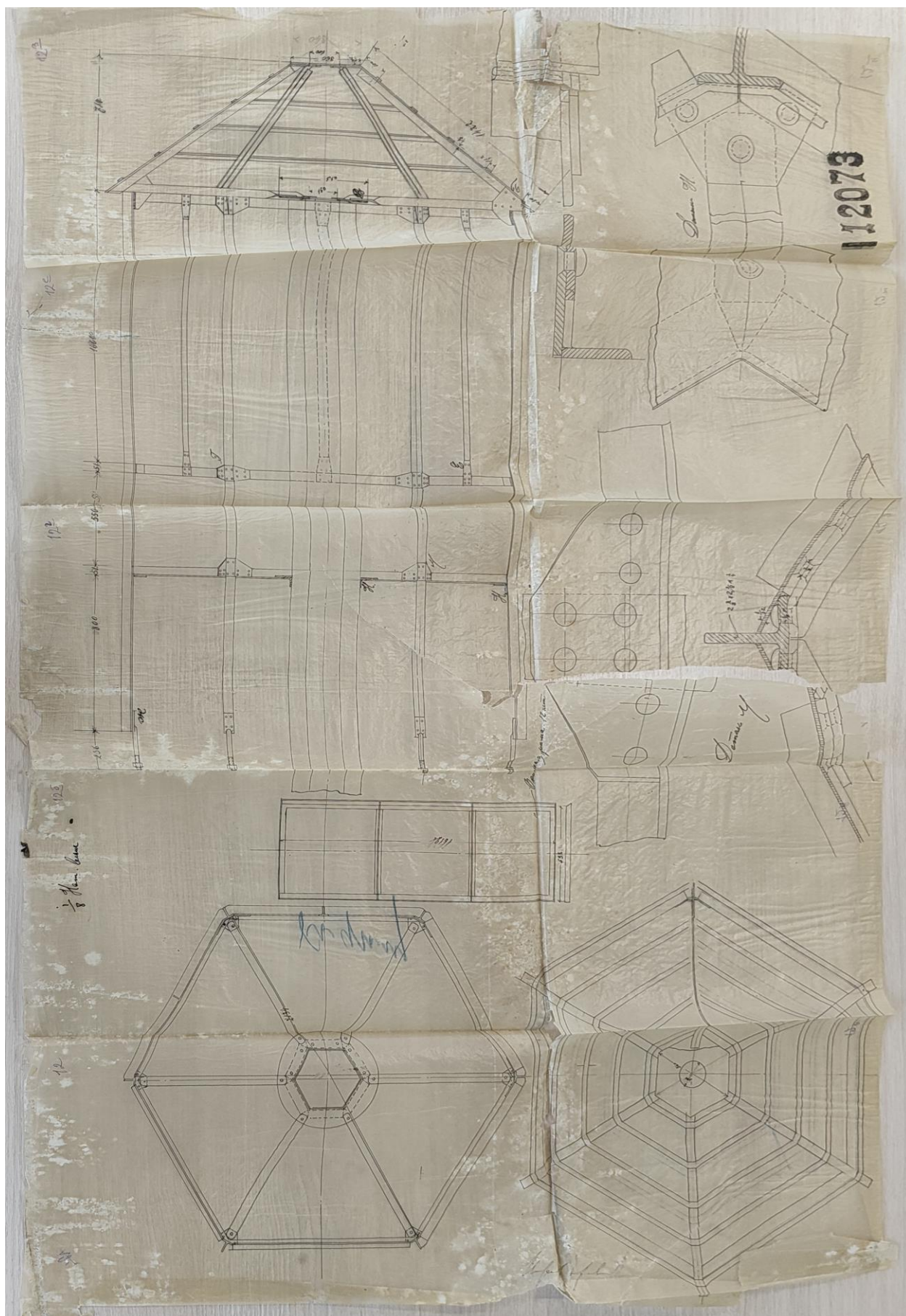
Илл. 23. Проект реконструкции башни Торпакова маяка. 1897 г. (источник: ЦГИА СПб. Ф. 921. Оп. 95. Д. 502).
