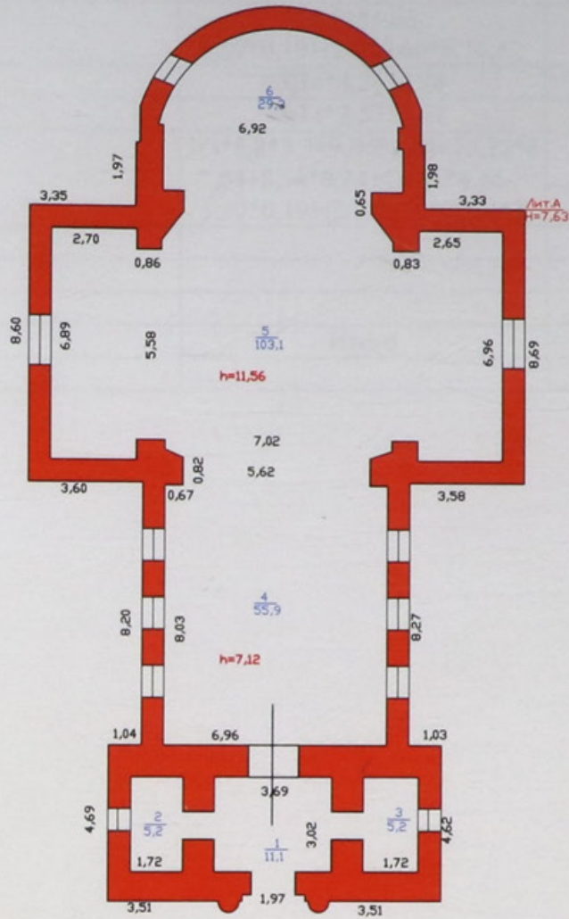
План 1 этажа
