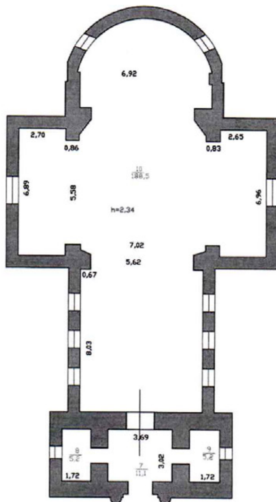
План подвала
