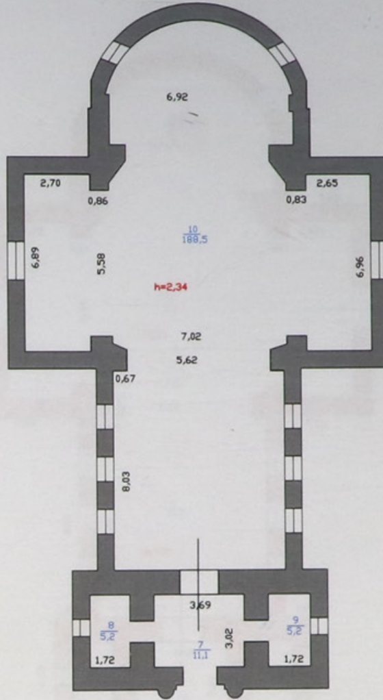
План подвала
