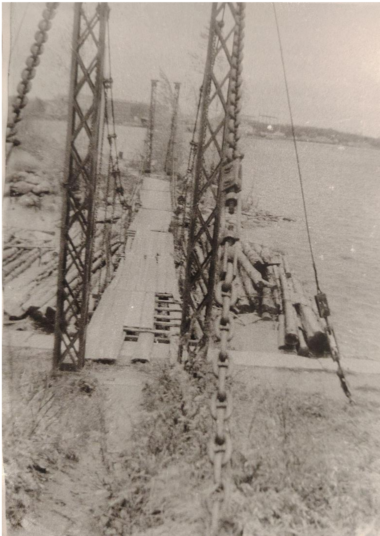
Илл. 13. Висячий мост на берегу Невы в зоне устья Петровского канала. Дата: 1984 г. Источник: архив Комитета по сохранению культурного наследия Ленинградской области (1614-2, инв. 5174).
