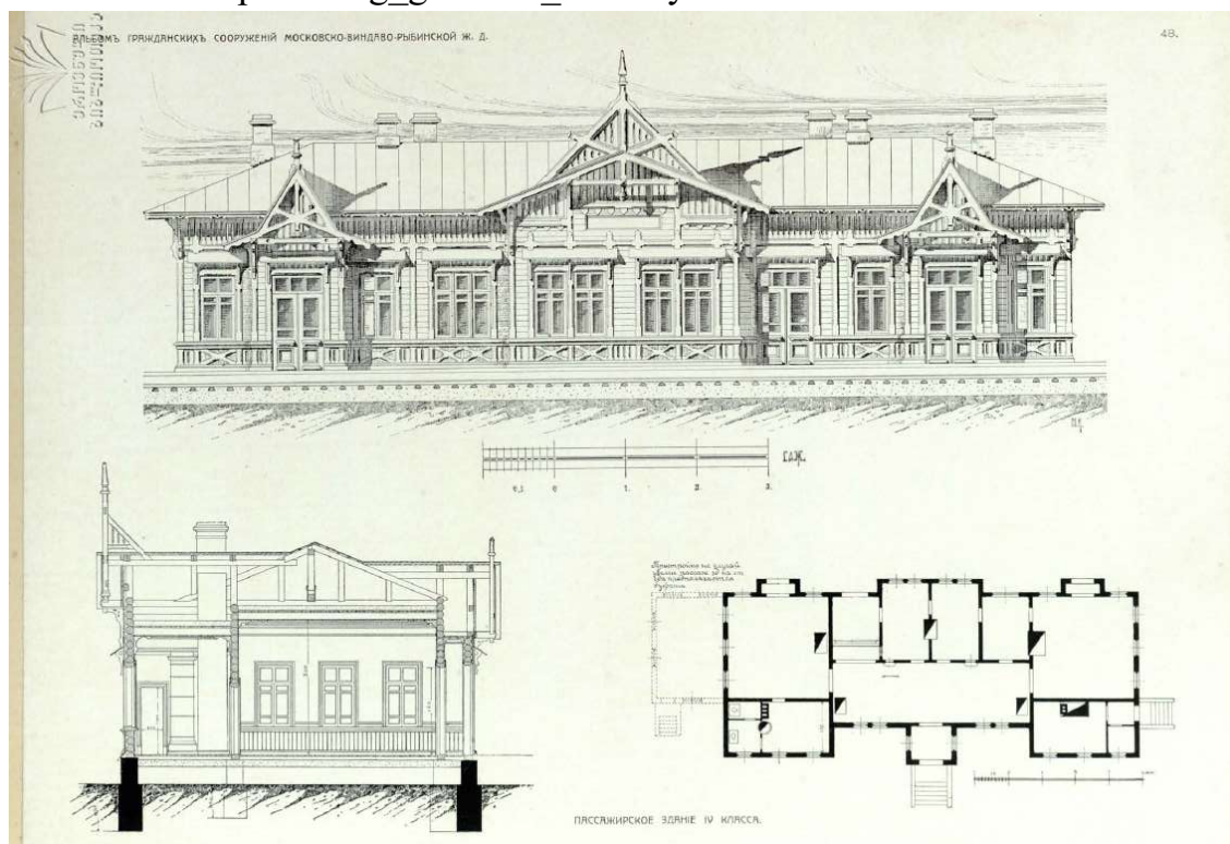
6. Пассажирское здание 4 класса. Альбом гражданских сооружений Московско-Виндаво-Рыбинской железной дороги. 1909
