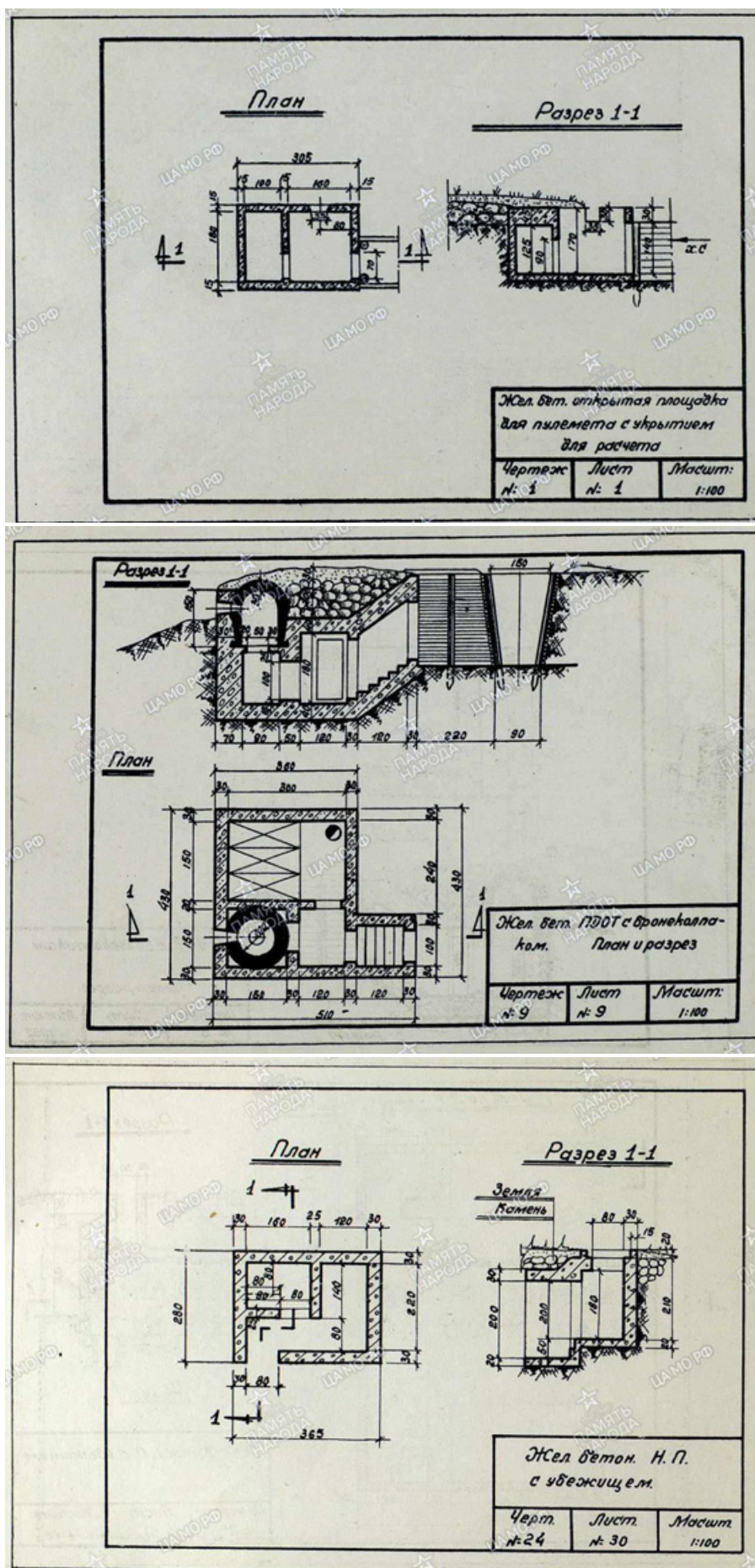
Илл. 39. Чертежи фортсооружений второго оборонительного рубежа финнов на Карельском перешейке. Варианты. 1944 г. [Электронный ресурс] // URL: https://www.photo.aroundspb.ru/fortification/vt-linja/ .
