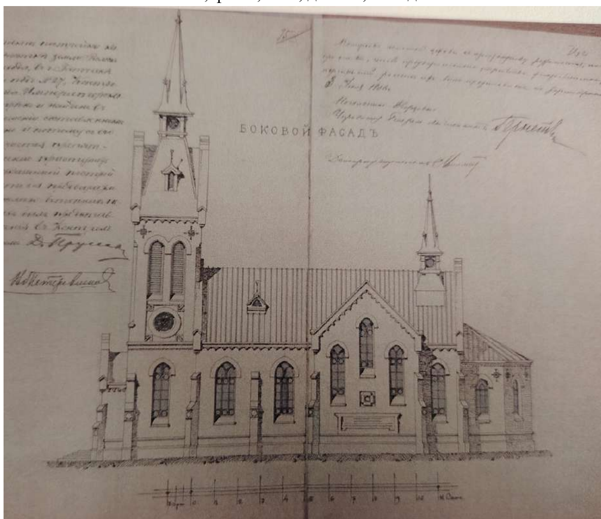
11. Проект каменного костела. Л. Шишко. Боковой фасад. РГИА, ф.491,
