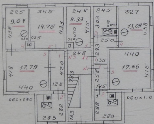
План 1 этажа
