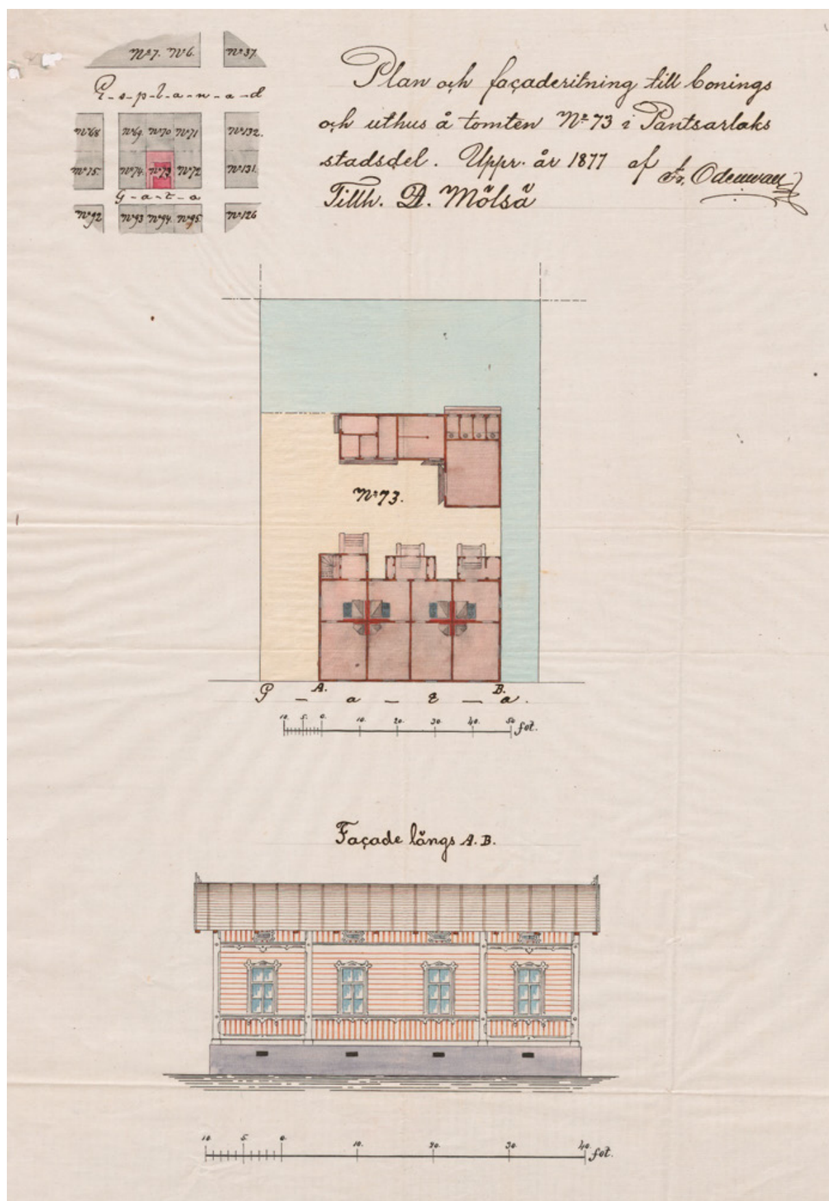
Илл. 78. План и фасад построек на участке № 73 в Панцарлах. Владелец Д. Мелся (D. Mölsä). 1877 г. Авт. Фр. Оденваль. Идент. 2550. [Электронный портал] URL: https://astia.narc.fi/uusiastia/viewer/?fileId=&aaineistoId=1677842827 .
