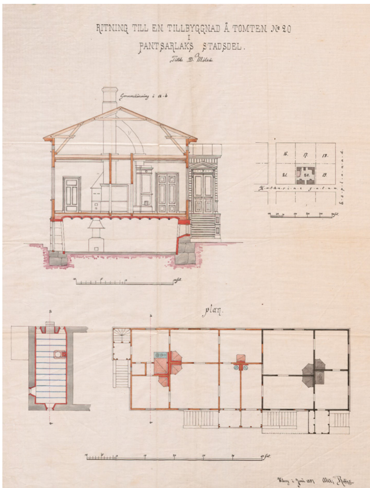
Илл. 35. Чертеж пристройки к зданию на участке № 20 в Панцарлах. Владелец Д. Мелся (D. Mölsä). 1887 г. Авт. Алекс. Рутин. Идент. 2084. [Электронный портал] URL: https://astia.narc.fi/uusiastia/viewer/?fileId=&aineistoId=1677002432# .
