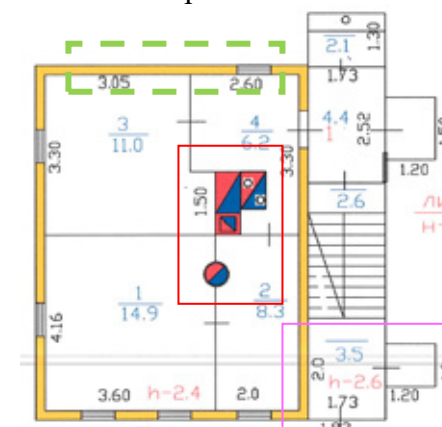
План 1-го и 2-го этажа. 2009 г.
