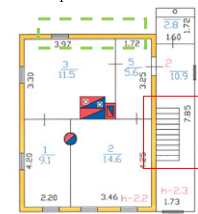
План 1-го и 2-го этажа. 2009 г.
