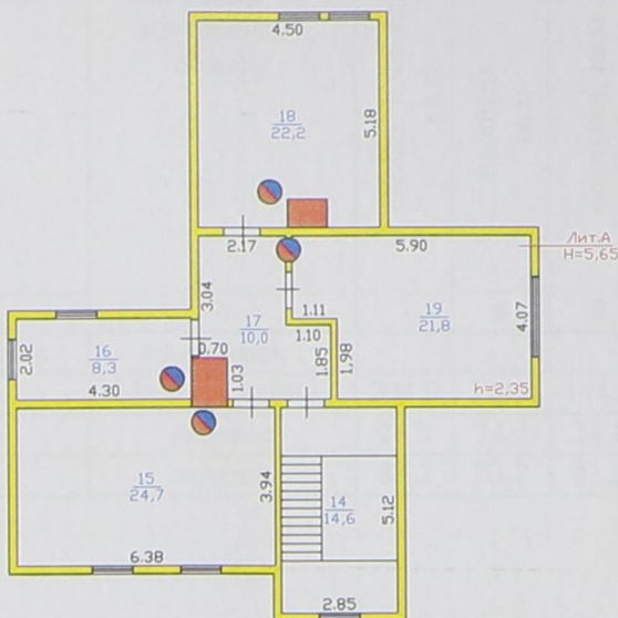
План 2 этажа
