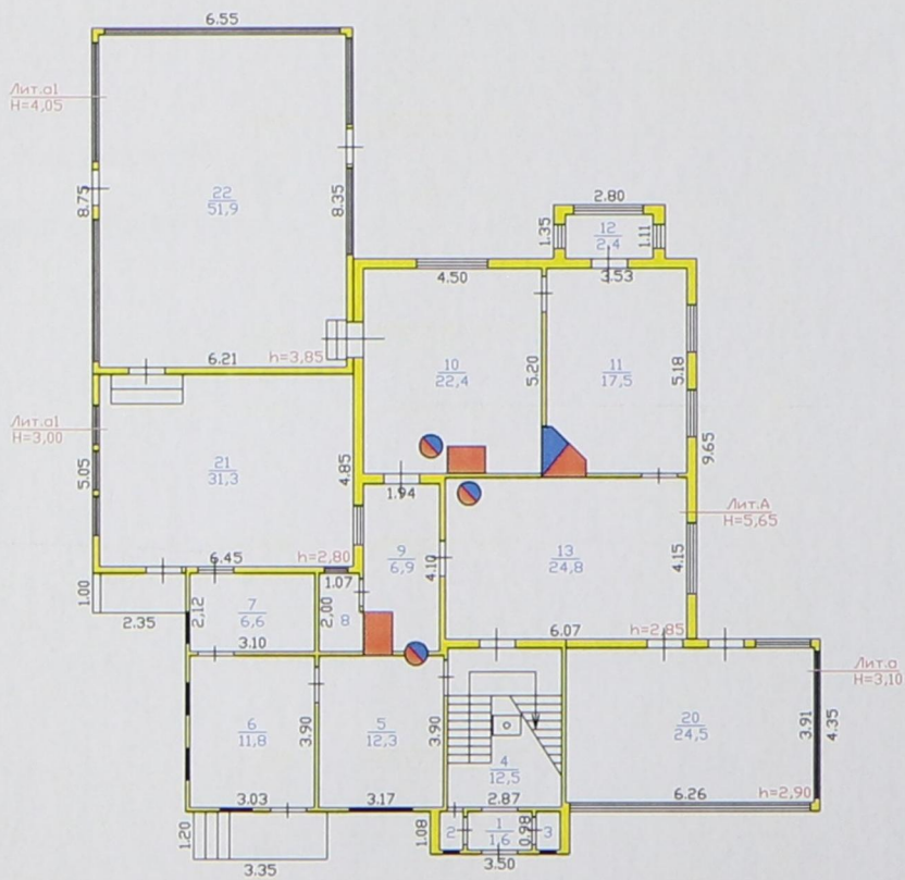
План 1 этажа
