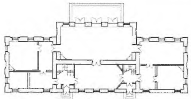
План 1-го этажа
