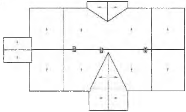
План кровли
