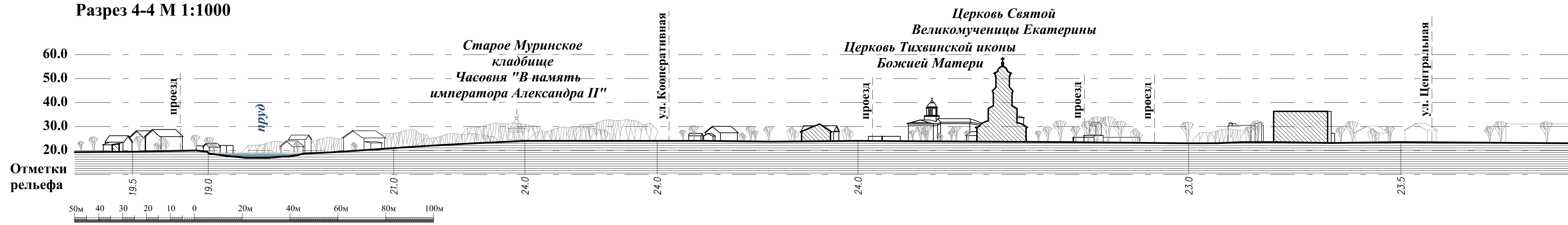
Разрез 4-4 М 1:1000
