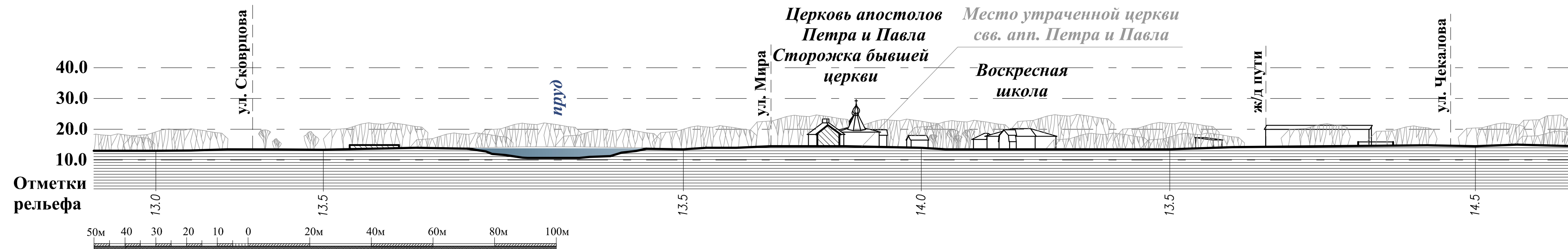
Разрез 2-2 М 1:1000
