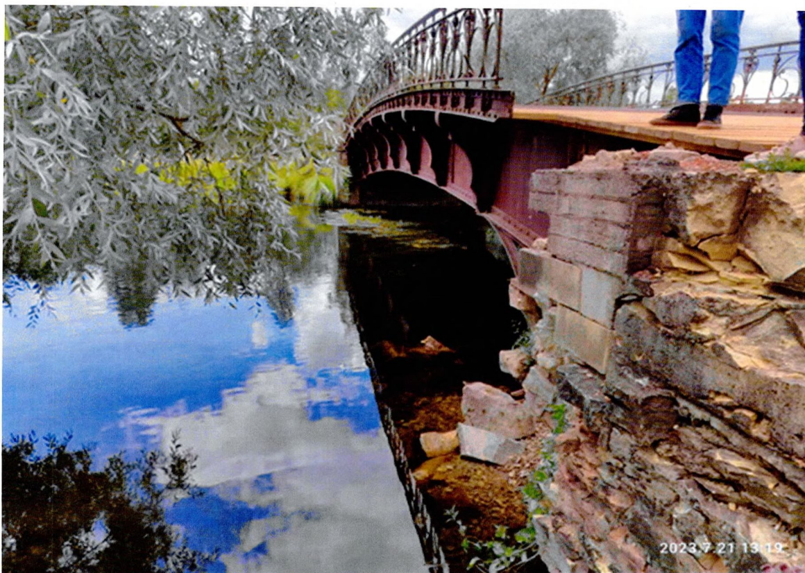
Фото 9. «Осиновый мост». Вид с правого берега по верховой стороне, зафиксированы вывалы каменных рядовых и карнизных блоков, обрушения каменной тумбы на устое.
