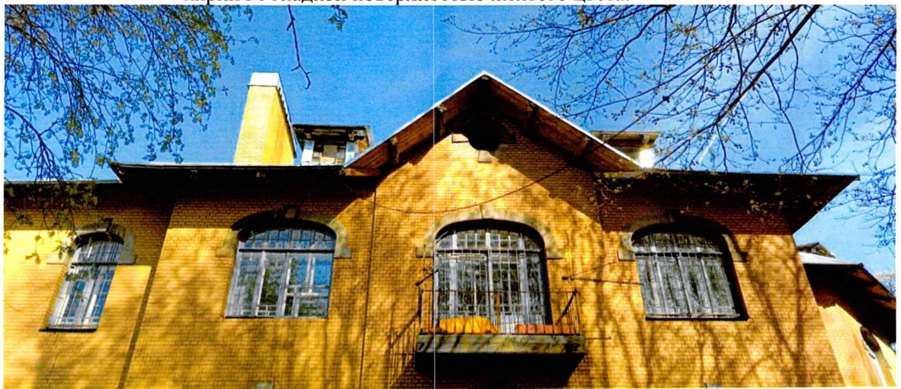
Фото 2. Фрагмент западного фасада. Вид в уровень 2 этажа.
