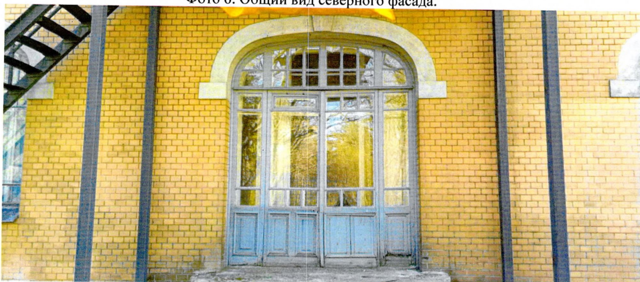
Фото 7. Историческое заполнение проема восточного входа – деревянное с многочастной расстекловкой и филенками в нижней части (предмет охраны).
