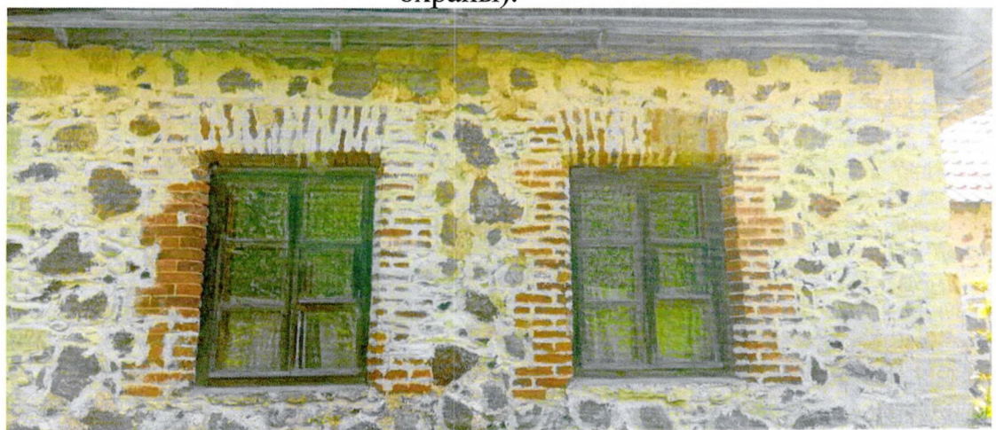
Фото 2. Оконные проемы ризалита западного фасада. Стены выполнены из крупных гранитных валунов, оконные проемы обрамлены кирпичной кладкой. Углы здания выполнены из обработанных каменных блоков (предмет охраны).
