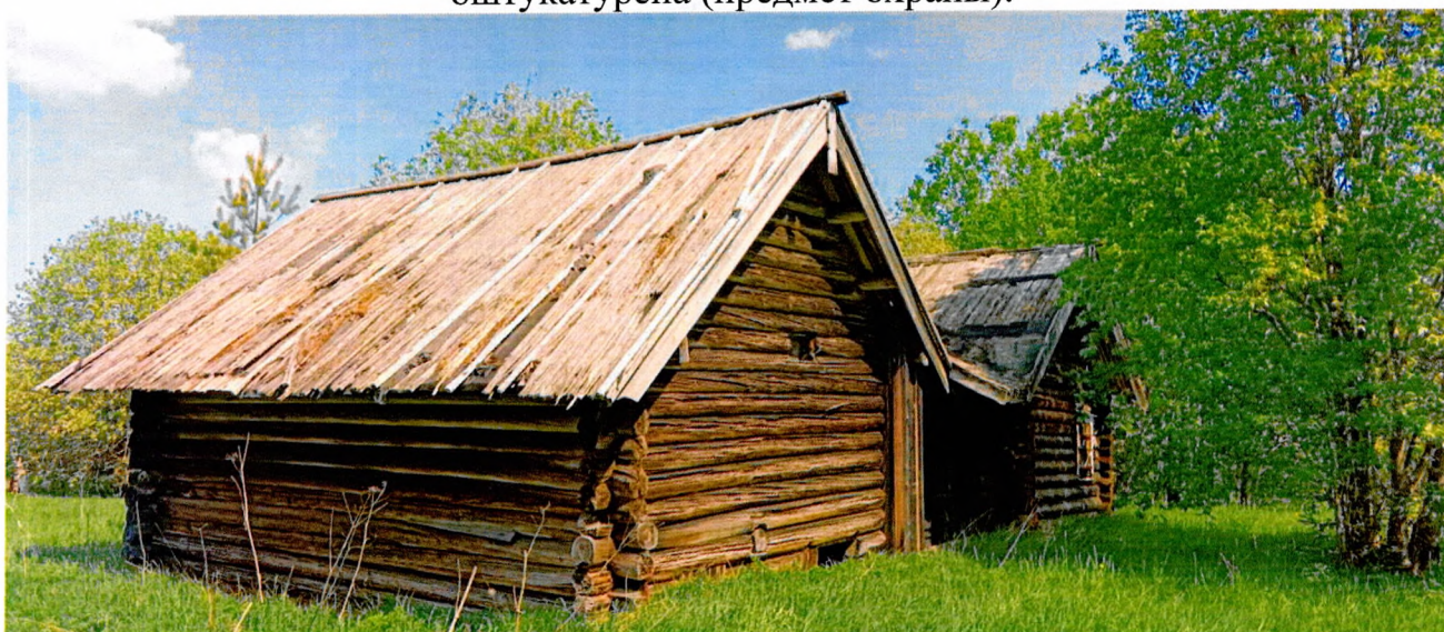
Фото 8. Общий вид с юго-запада. Строение представляет собой два объема – жилой и хозяйственный – прямоугольных в плане, покрытые двускатной кровлей и соединенные сенями.
