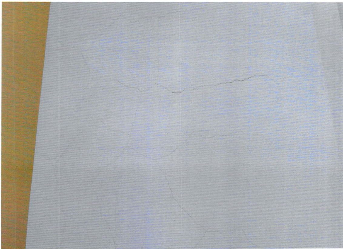
Фото 5. Фрагмент западного фасада. Сетки трещин на колоннах.
