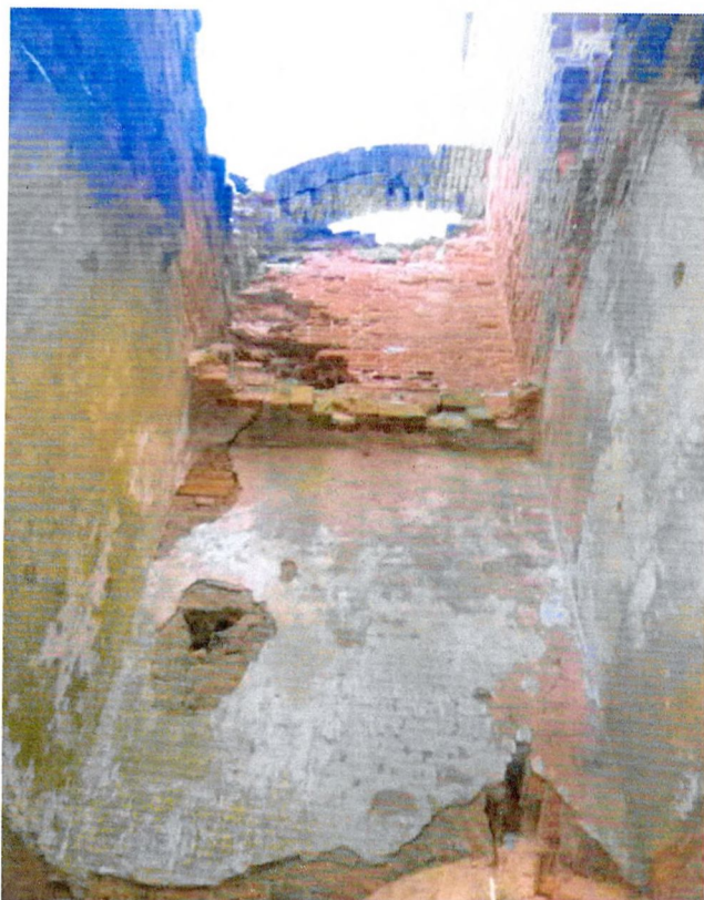
Фото 38. Биоповреждения штукатурного слоя в приделе северной части здания.
