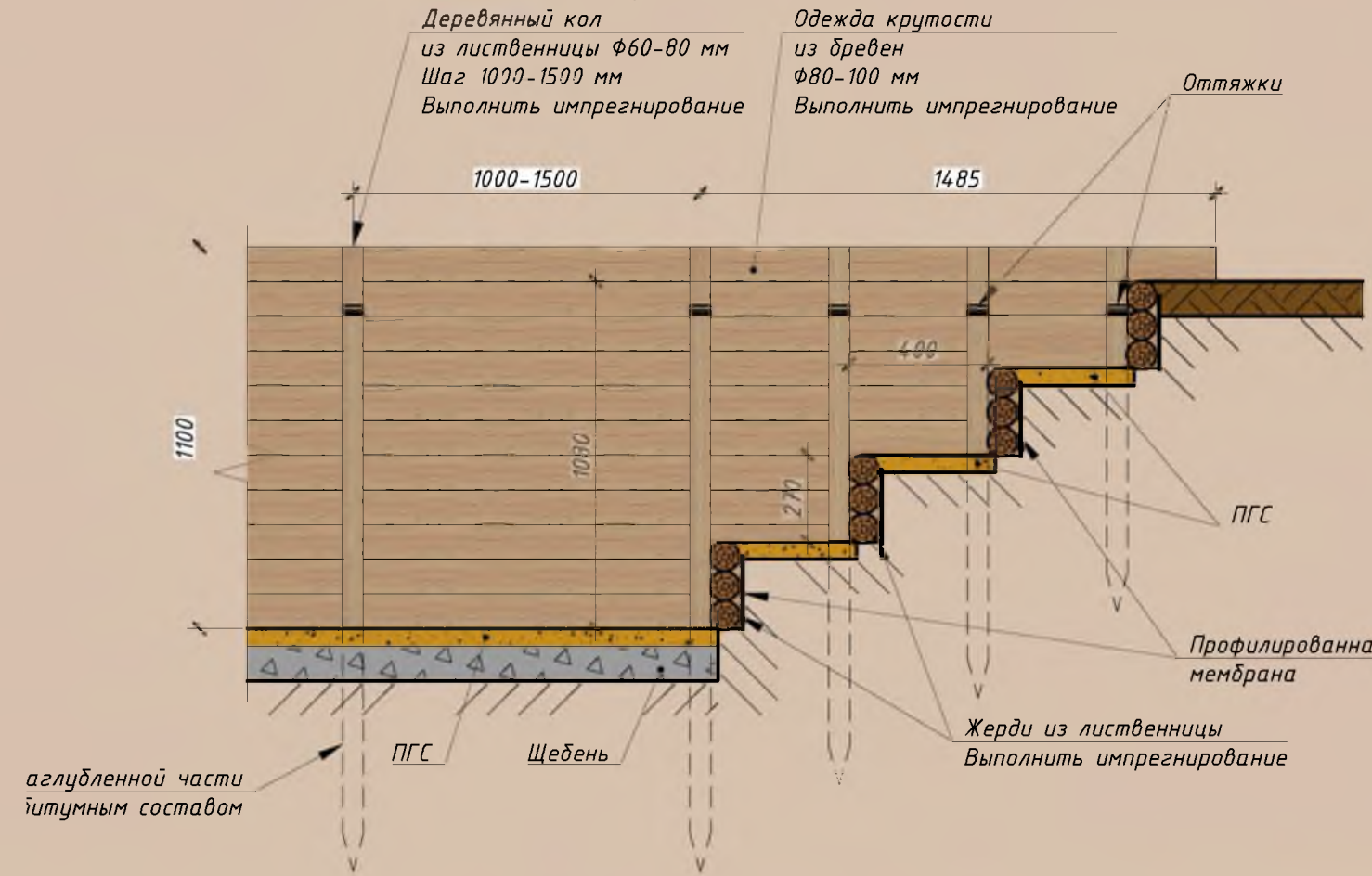
Разрез 3-3
