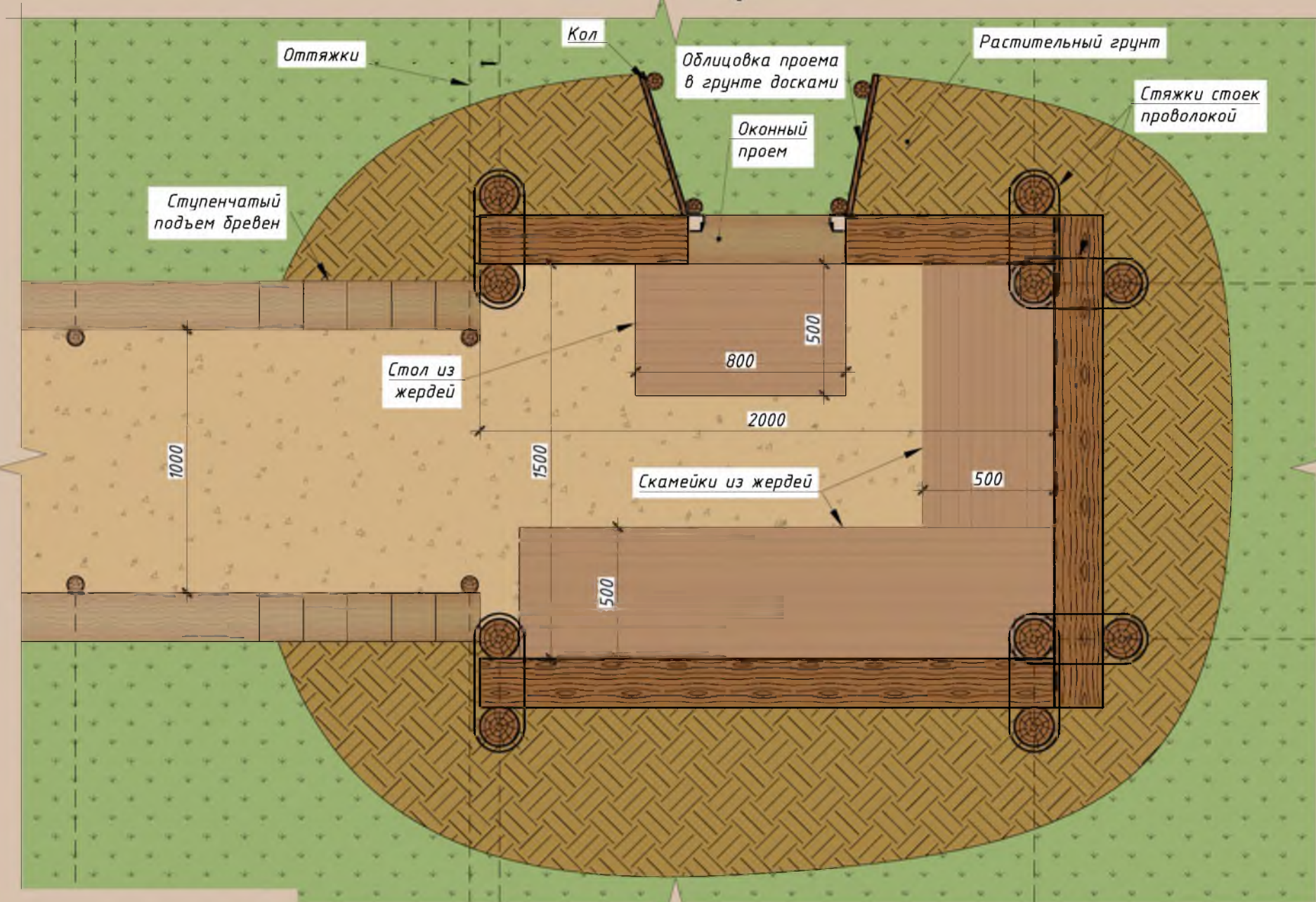
План блиндажа
