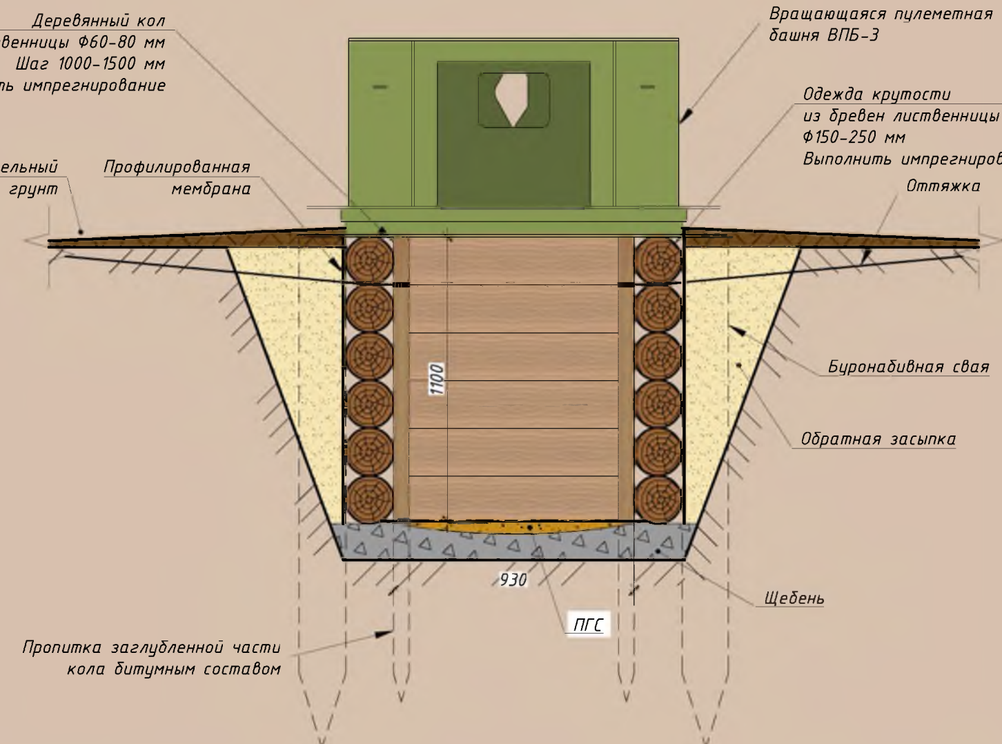
Разрез 5-5
