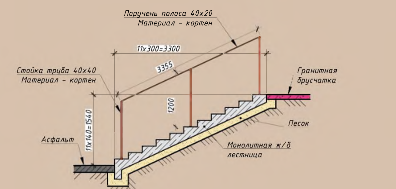
Разрез 2-2
