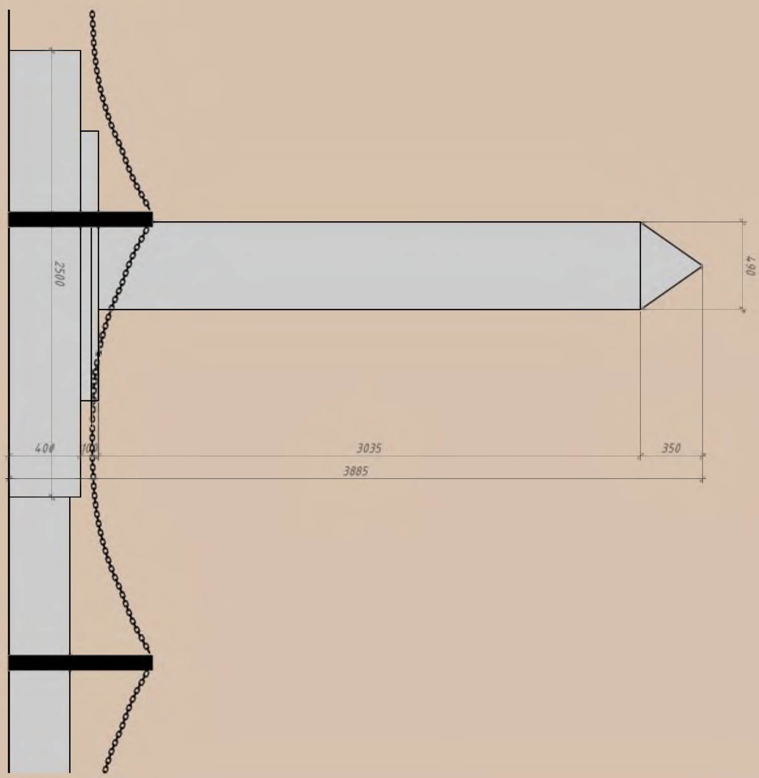
Стела. Боковой фасад
