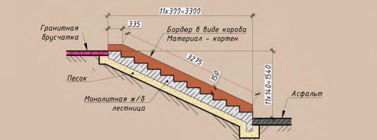
Разрез 2-2
