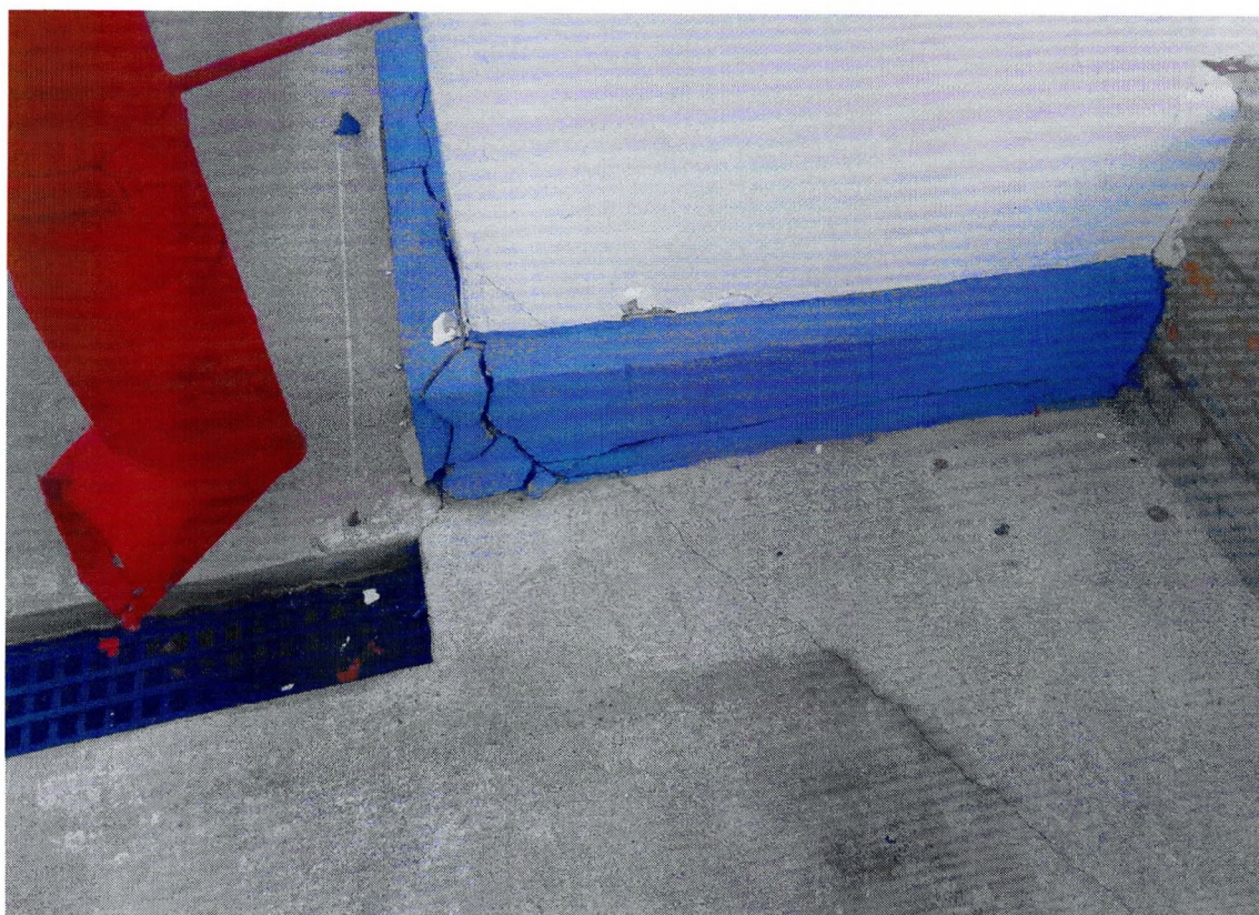
Фото 4. Фрагмент южного фасада. Растрескивание штукатурного слоя цоколя. Трещина в бетонной отмостке.
