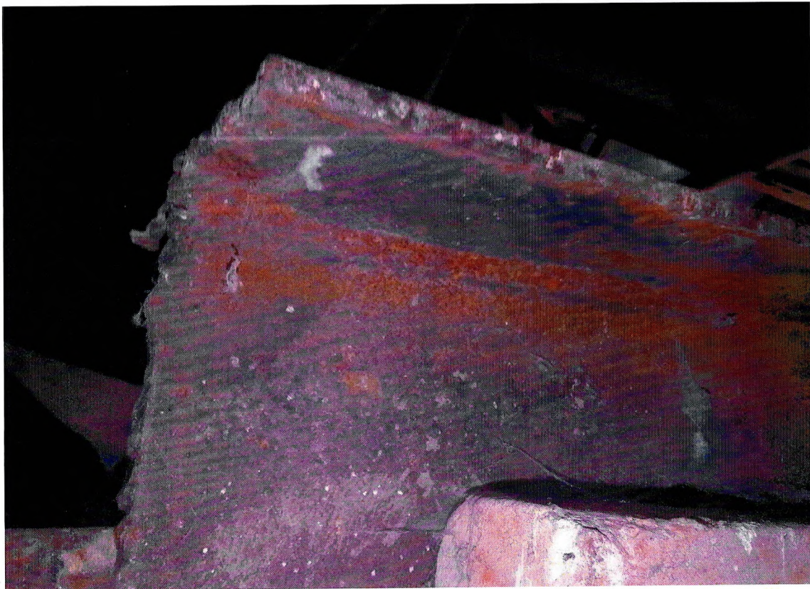
Фото 21. Коррозия металлической чердачной балки.
