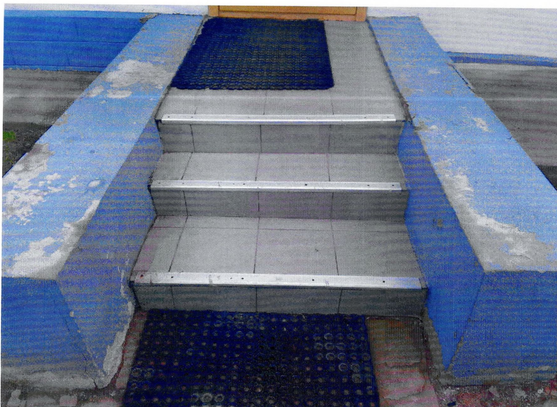
Фото 11. Фрагмент западного фасада. Отслоение штукатурного слоя крыльца.
