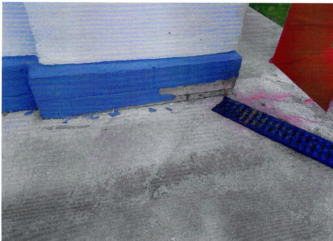
Фото 6. Фрагмент южного фасада. Отслоение штукатурного слоя цоколя.
