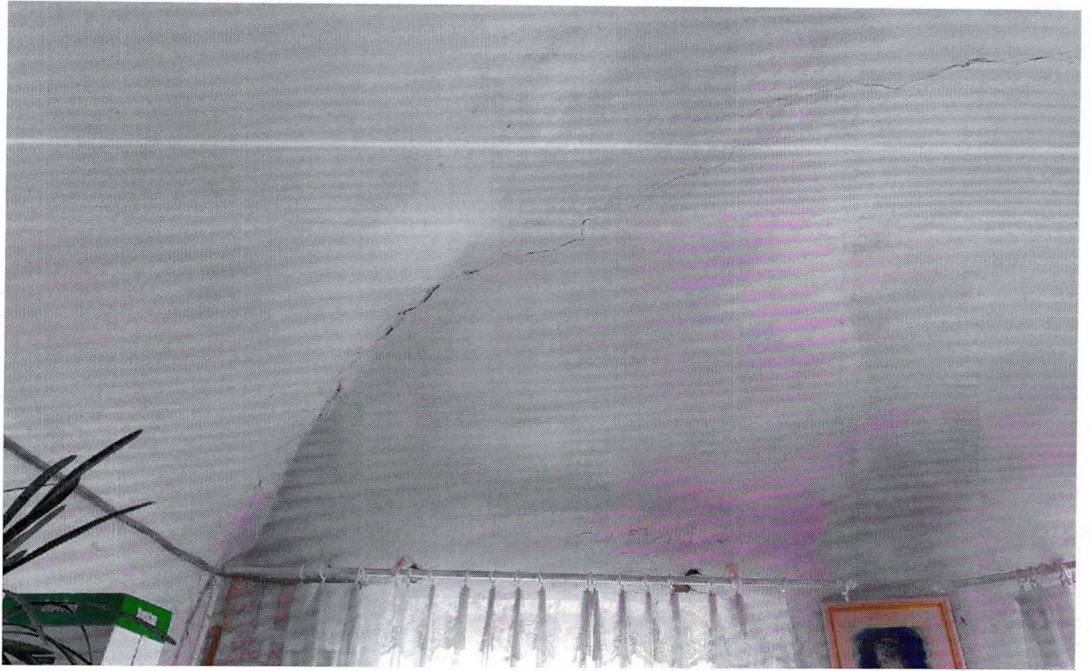
Фото 25. Трещины отделочных слоев во внутреннем помещении первого этажа
