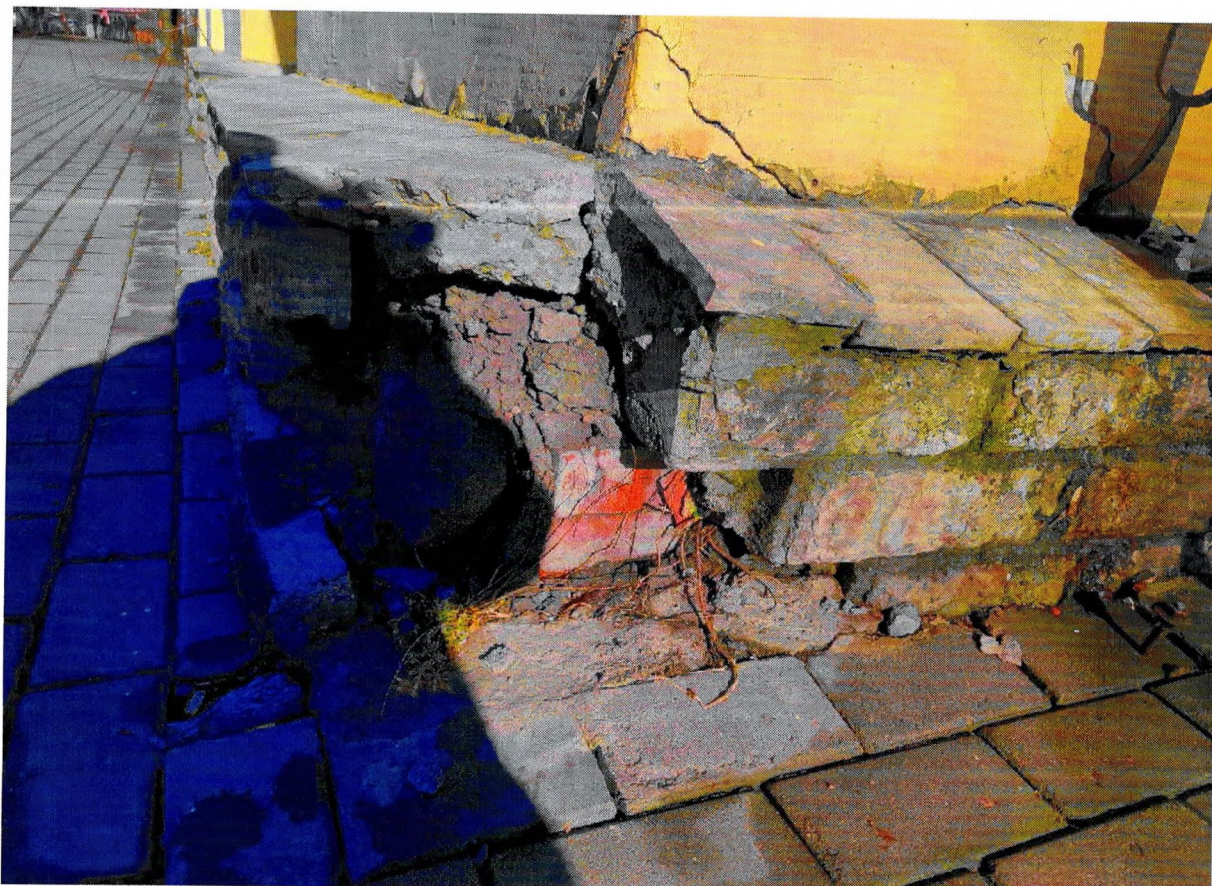
Фото 5. Фрагмент южного фасада: утрата облицовки цоколя на углу здания, трещина штукатурного слоя
