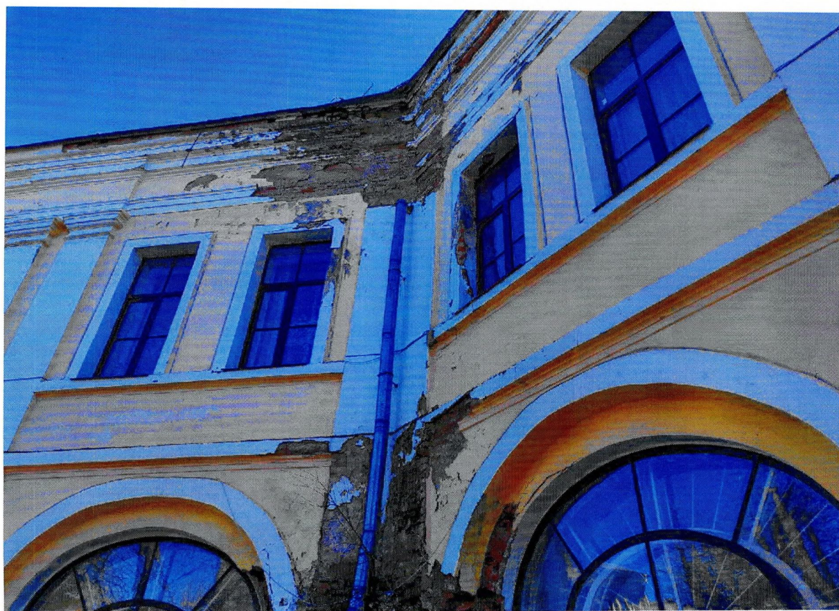
Фото 8. Фрагмент юго-западного фасада: разрушения штукатурки и части декоративных элементов, утрата части водосточной трубы
