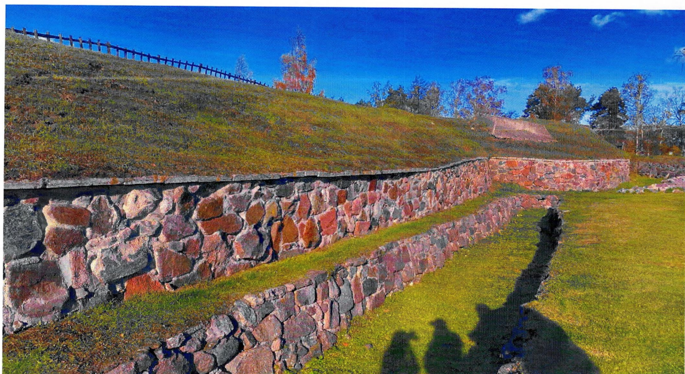
Фото 20. Общий вид на Басту бастион, Теналь и канал на территории
