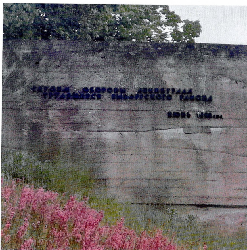
Фото 40. Внешняя стенка второй смотровой площадки, с надписью. Поверхность бетона сильно загрязнена, имеет биопоражения. Разрушение защитного слоя бетона, отслоение и трещины. В нижней части стены отсутствует верхний слой с опалубкой.
