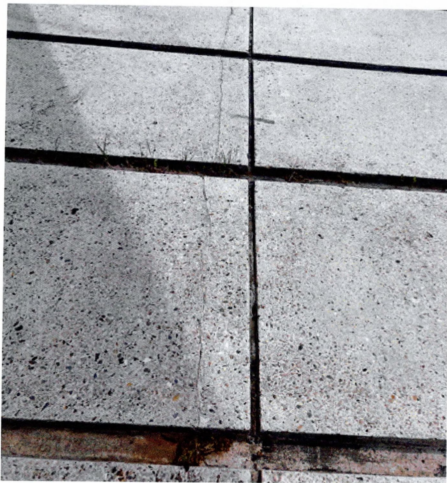
Фото 7. Фрагмент бетонной плиты стилобата с покрытием «террацо». Трещины в плитах покрытия, в желобах между плитами самосевная растительность.
