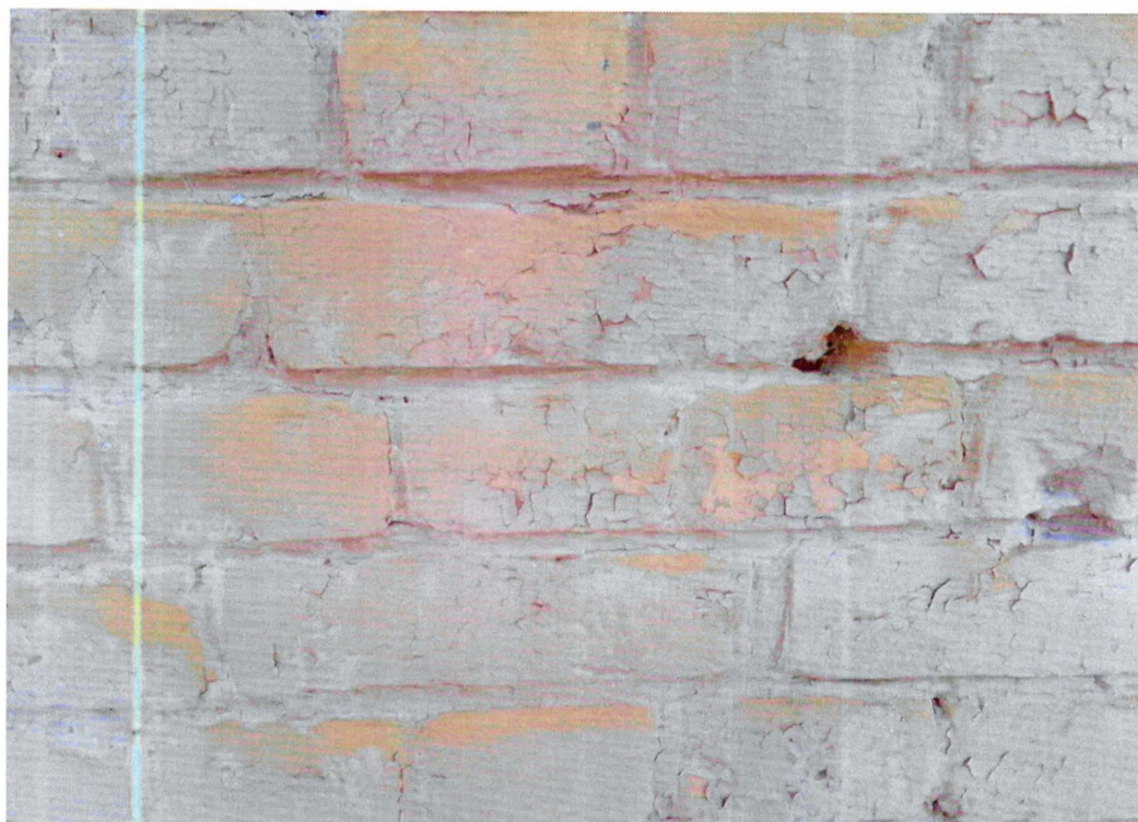
Фото 4. Фрагмент западного фасада. Шелушение окрасочного слоя неоштукатуренной поверхности стен фасада.
