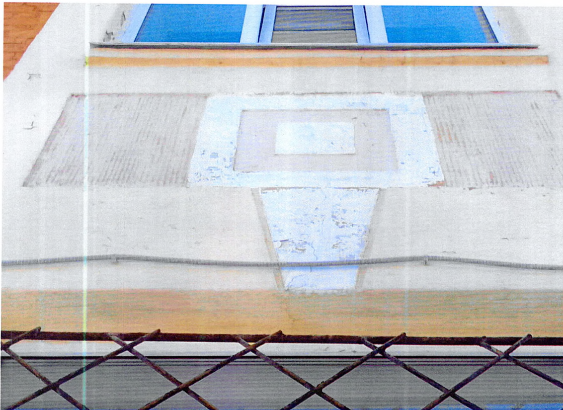
Фото 5. Фрагмент западного фасада. Трещины в штукатурном слое.
