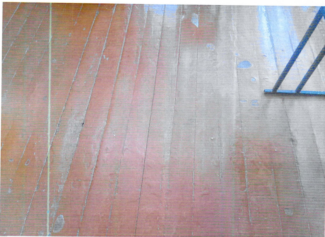
Фото 29. Стирание досок в ходовых местах, сколы досок местами, повреждения отдельных досок дощатых полов.
