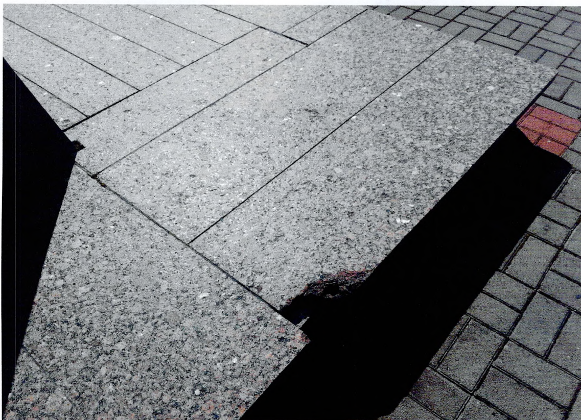
Фото 4. Скульптура партизана. Скол гранитной плиты, утрата шовного раствора между плитами.
