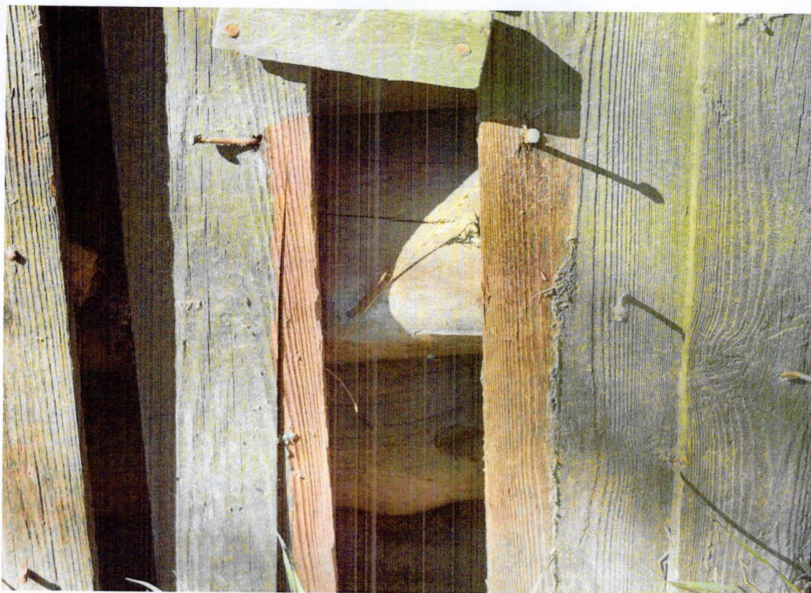
Фото 13. Фрагмент восточного фасада. В местах утрат обшивки фасада просматриваются бревенчатые стены.
