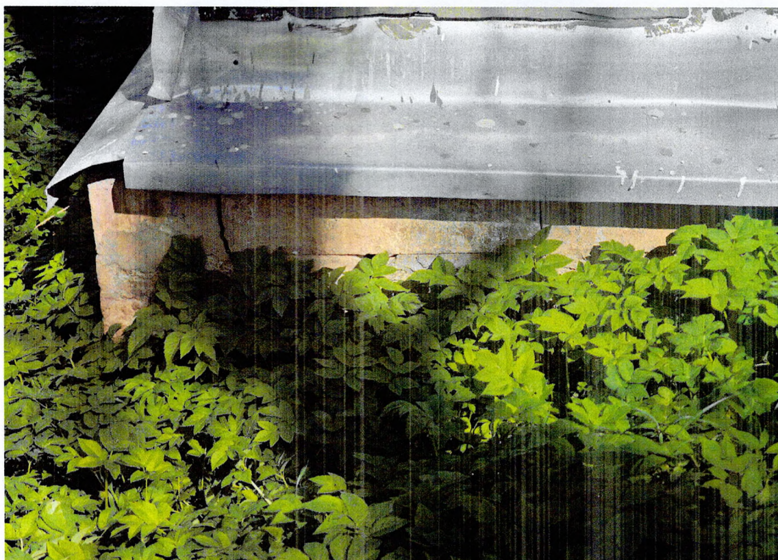
Фото 20. Фрагмент южного фасада. Каменный цоколь. Разрушение и осадка угла цоколя.
