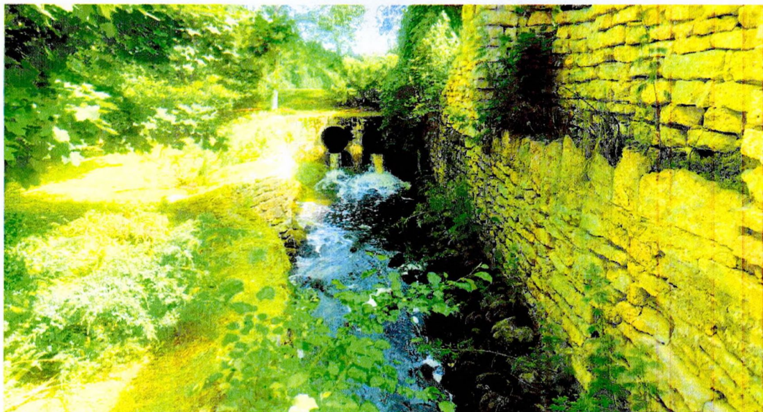
Фото 1. Вид на фрагмент северного фасада. Материал – обработанные каменные блоки. Шовное заполнение утрачено. Наблюдаются сколы на поверхности каменных блоков. Отмостка утрачена.
